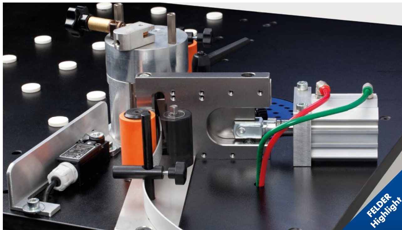
Prédécoupe pneumatique pour un usinage de haute qualité des chants droits et galbés
