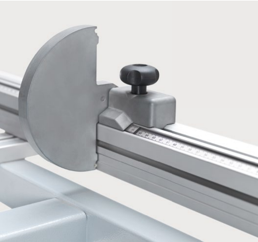
Anschlagsskala Die Skala der Ablänganschlüge ist zur Bedienseite hin geneigt und erleichtert so das exakte Ablesen des gewünschten Einstellwertes.
