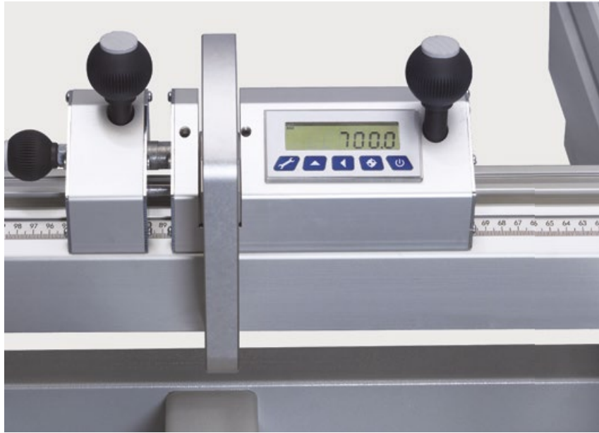
Ablänganschlagbacken Auf Wunsch: Digitaler Ablänganschlagbacken für zehntelmillimetergenaue Einstellung.
