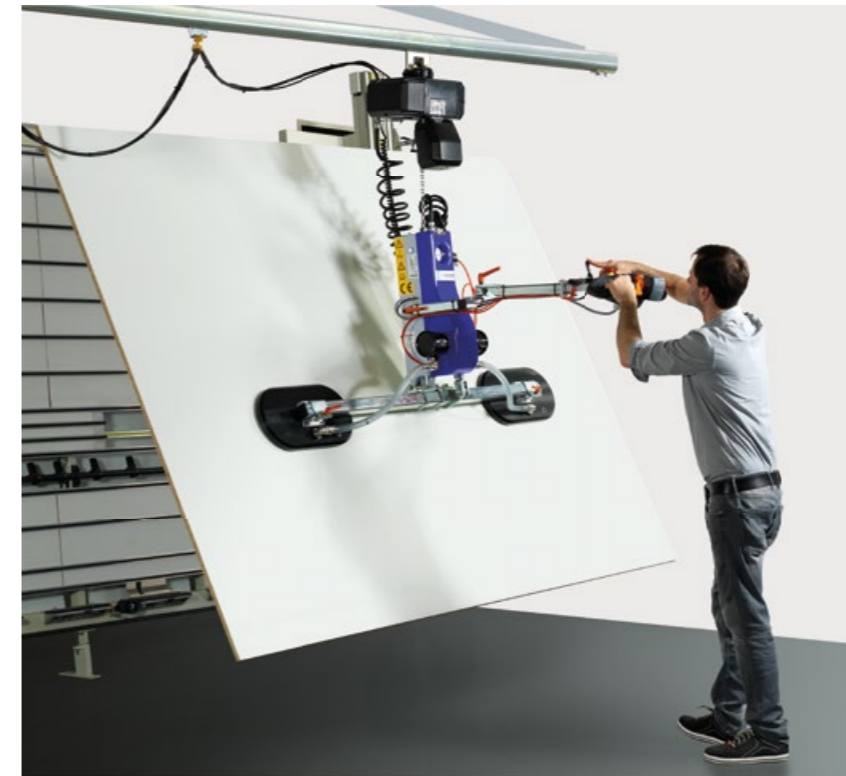
Anwendungsbild Das ideale Hilfsmittel für den schnellen und effizienten Transport von beschichteten Spanplatten! » Traglast 250 kg: v-motion classic » Traglast 150 kg: v-motion 15.00 » Traglast 150 kg: v-motion 15.90 » Traglast 200 kg: v-motion 20.90 » Traglast 250 kg: v-motion 25.90st » Säulenschwenkkran 4000 mm » Komfortbedienung für einfachstes Handling
