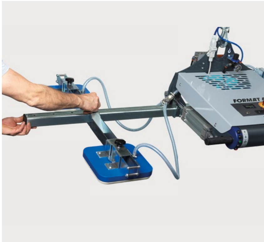
Verstärkte Saugtraverse für einen sicheren Plattentransport (v-motion 20.90 classic) 2 m Längstraverse mit 4 verstellbaren Saugtellern zu je 250 x 250 mm
