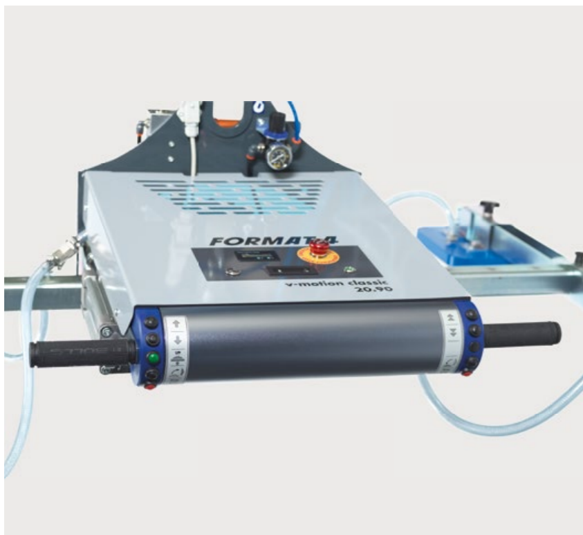
Innovative Bediensteuerung für ergonomisches Plattenthandling (v-motion 20.90 classic) Einfache und intuitive Bedienung mit extra breitem Bedienterminal für mehr Präzision beim Plattentransport
