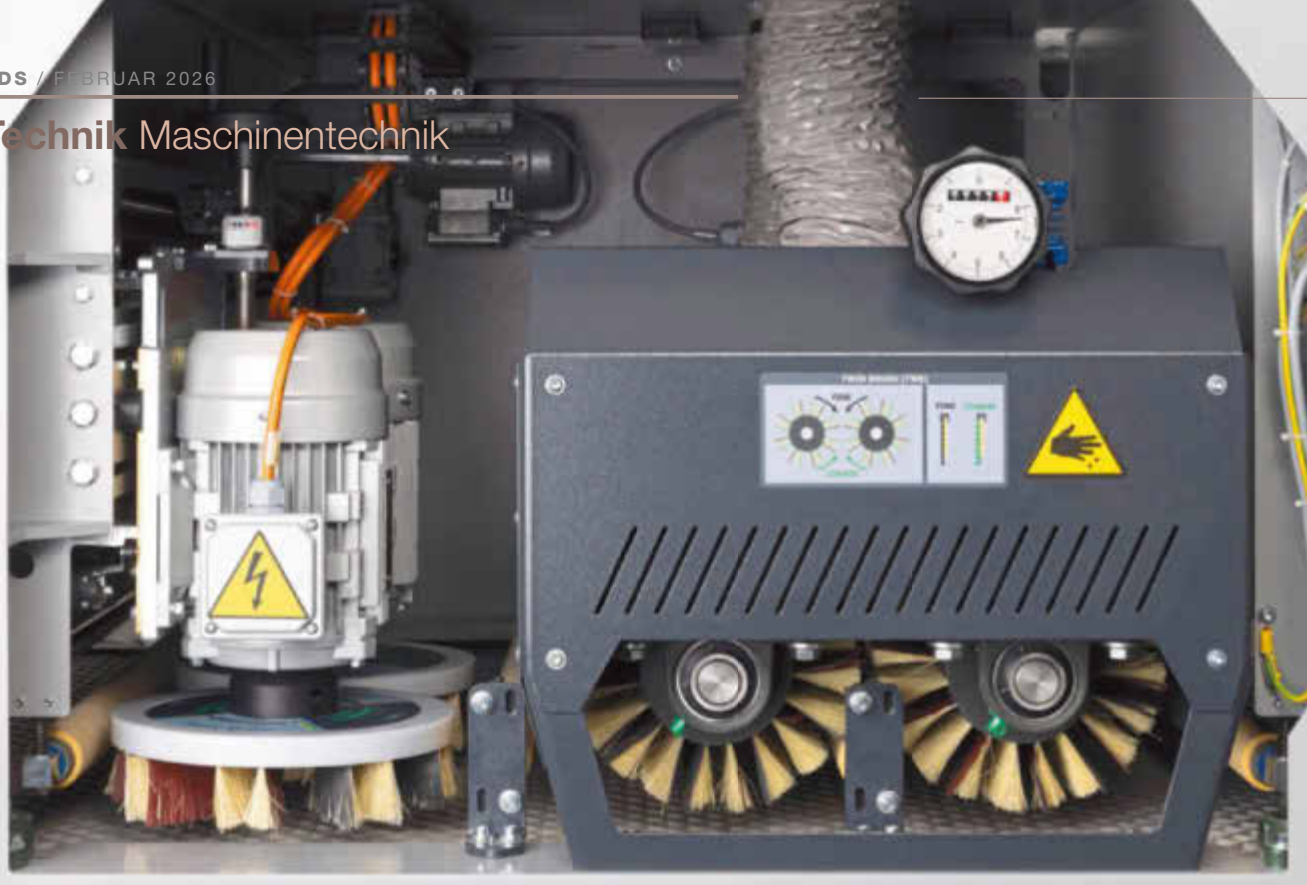
Zwei gegenläufig arbeitende Längsbürsten sowie ein Tellerbürstenaggregat erzeugen ein hervorragendes Finish
