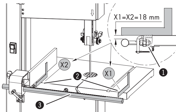
Att. 7-8: Augstuma iestatījums - Lineāla slīdes
