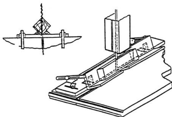
Att. 8-18: Šķēsgriezums
