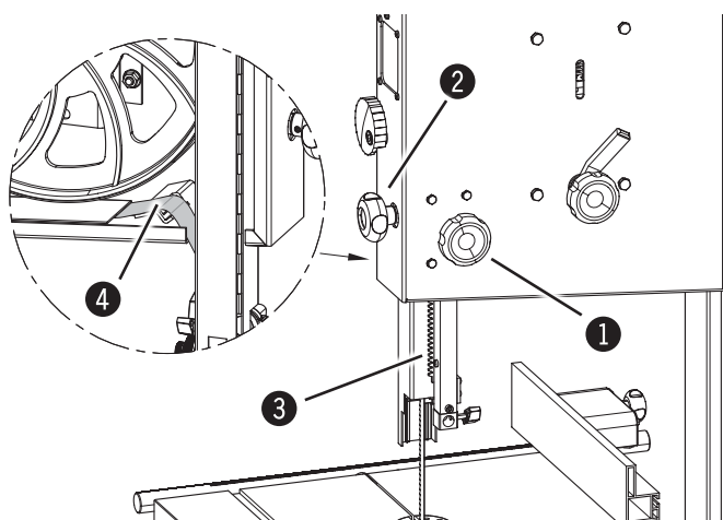
Att. 9-5: Regulējums - Zāglentes spriegojums
