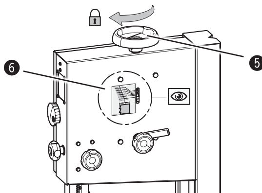
Att. 8-3: Zāģasmeņa nomaiņa
