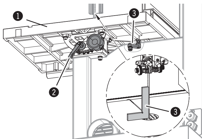
Att. 7-5: 90° zāglentes kustība
