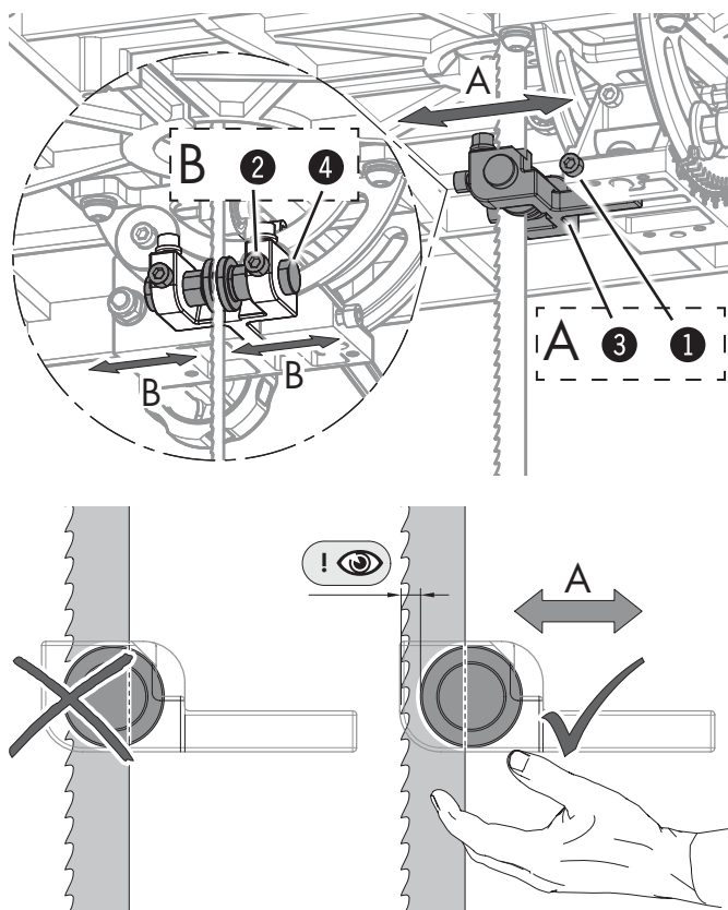
Att. 8-9: Vadotņu sāna elementu iestatīšana.
