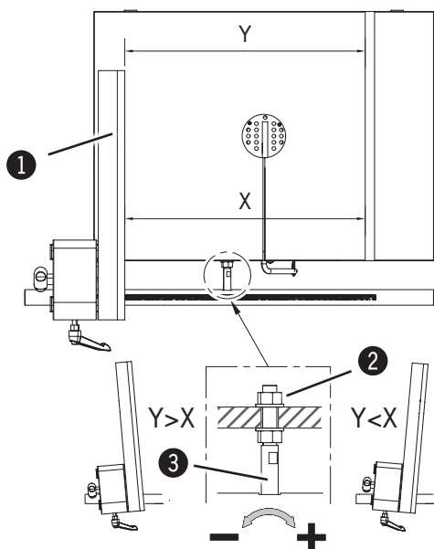
Att. 7-9: Paralēlā lineāla iestatīšana
