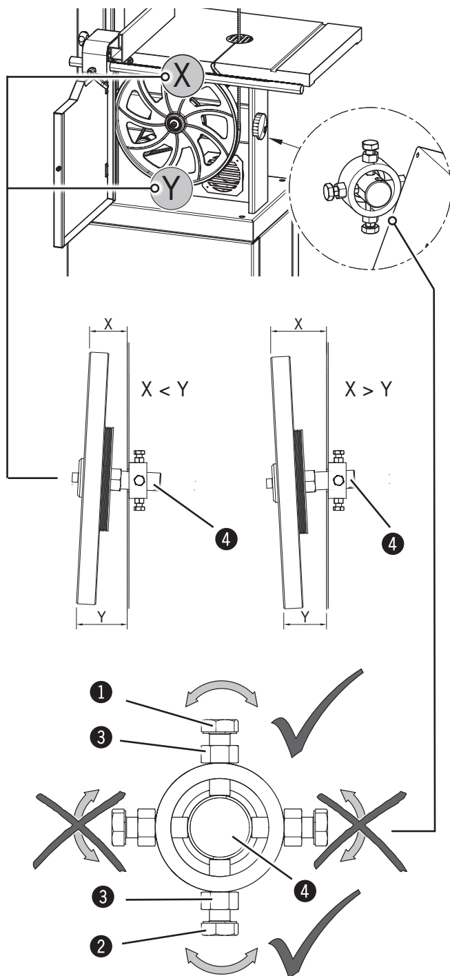
Att. 8-4: Iestatījumi - Zāgasmaņa ceļš/ Apakšējais rats
