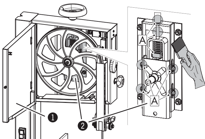
Att. 9-4: Regulējums - Zāglentes spriegojums
