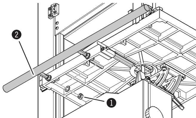
Att. 7-7: Paralēlās griešanas lineāls
