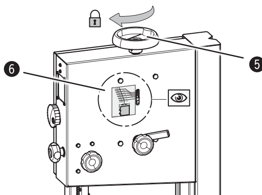
Fig. 7-3: Cambio de la hoja de sierra
