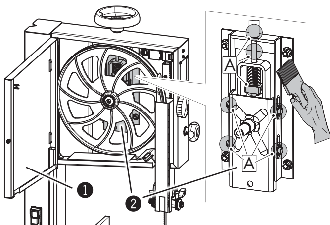
Fig. 9-4: Ajuste - Tensión de la hoja de sierra
