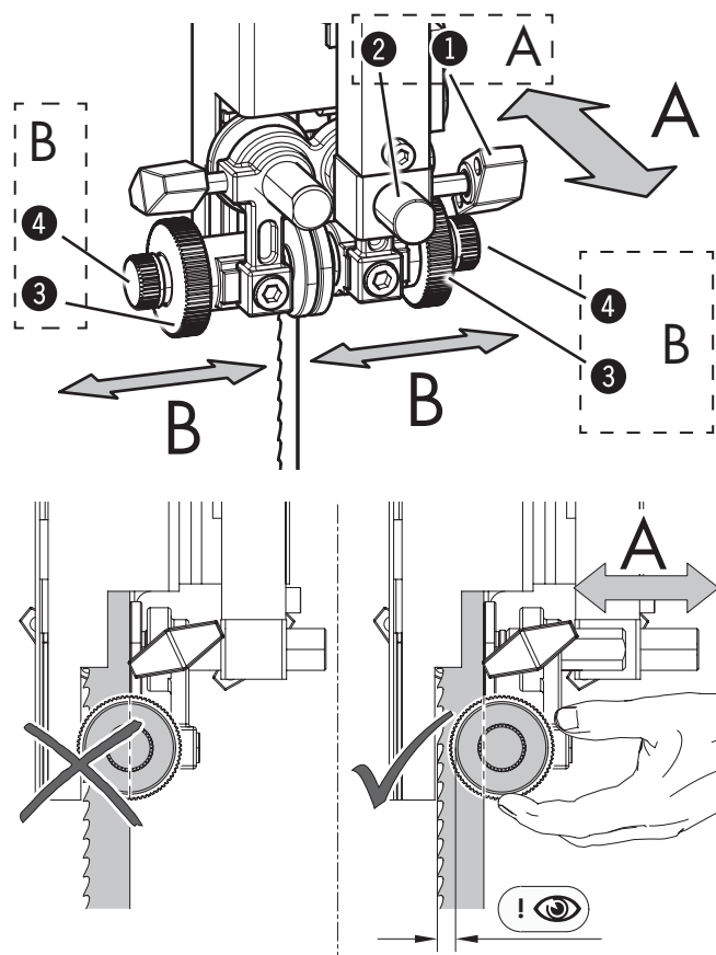
Fig. 8-7: Ajuste de los elementos de guía lateral
