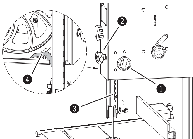
Afb. 9-5: Verplaatsing - Zaaglintspanning
