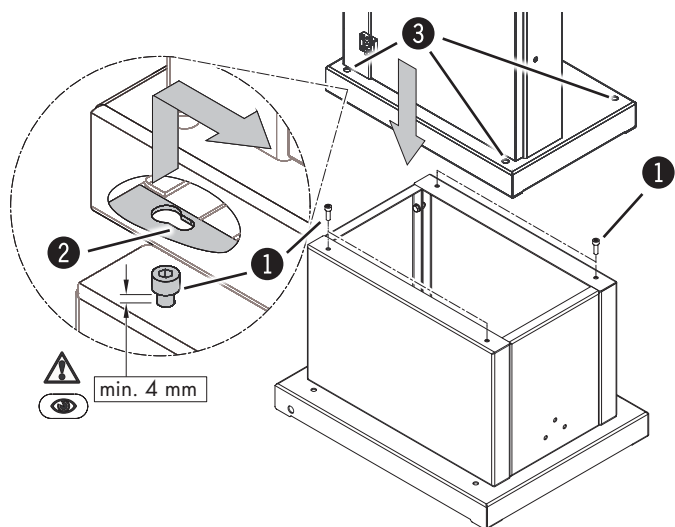
Afb. 7-3: Montage - Lintzaag
