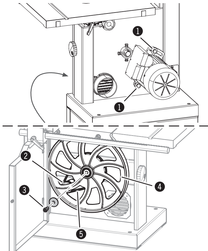
Afb. 9-2: Aandrijfriem vervangen
