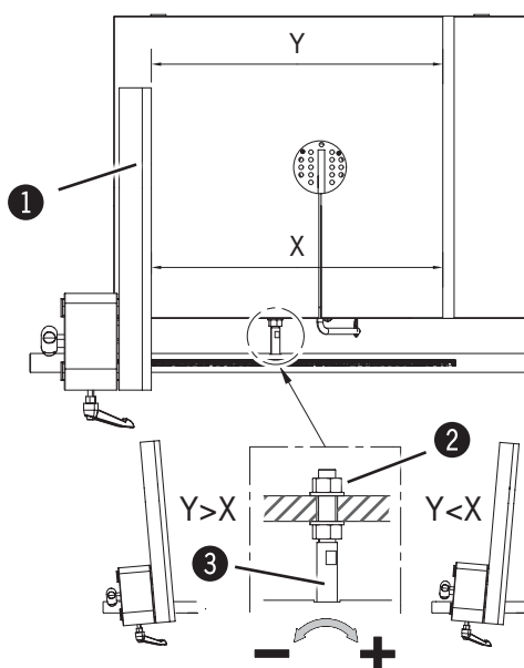
Afb. 7-9: Parallelaanslag instellen
