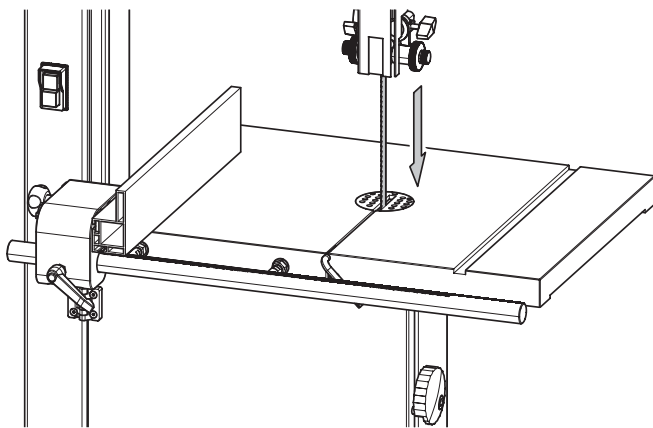
Afb. 7-11: Draairichting motor
