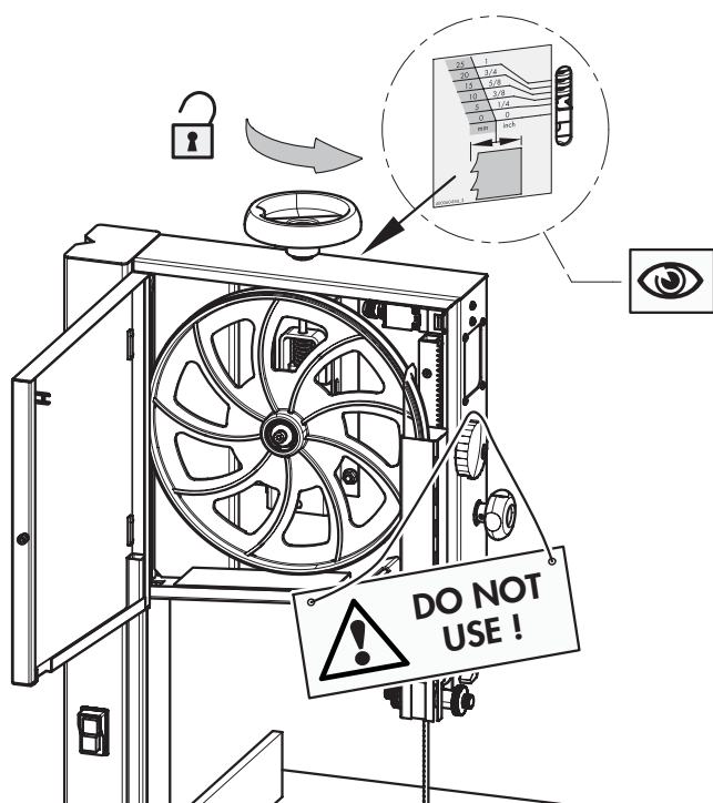
Fig. 8-2: Savklingspændingen løsnes
