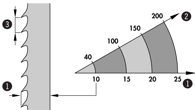
Fig. 8-1: Savklinger
