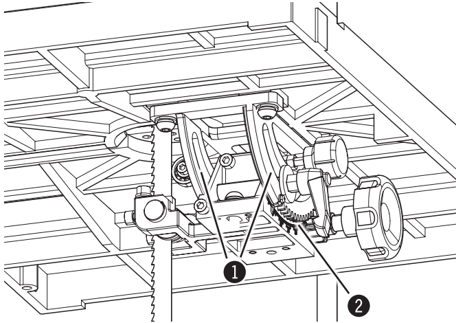
Fig. 9-6: Inclinazione piano
