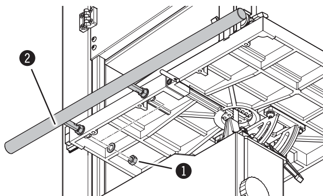
Fig. 7-7: Guida parallela
