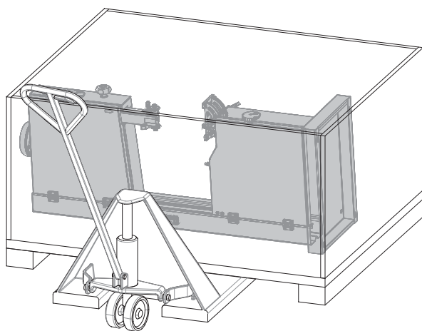
Ábra 6-1: Szállítási biztosítása
