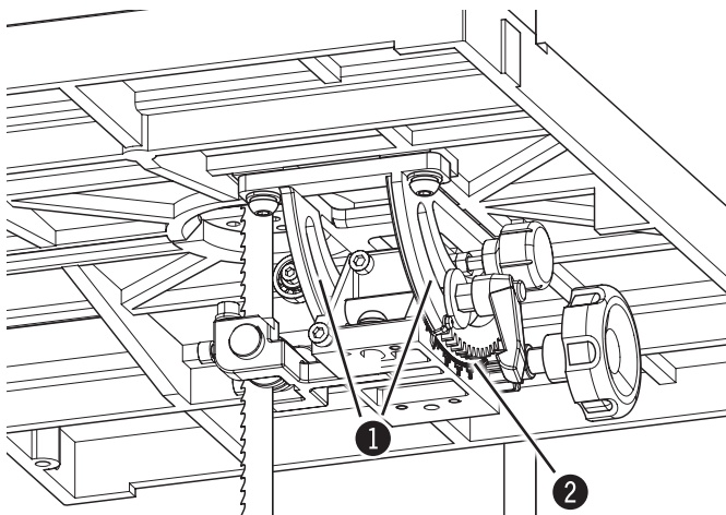
Ábra. 9-6: Asztaldöntő
