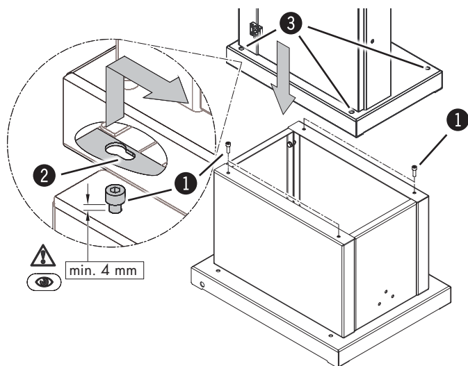
Ábra. 7-3: Szerelés - szalagfűrész
