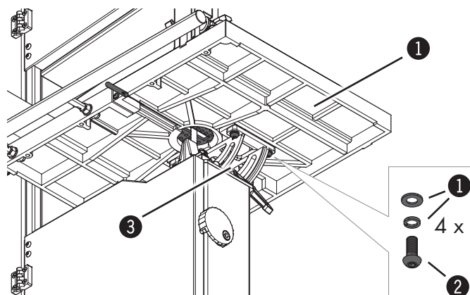
Ábra. 7-4: Munkasztal
