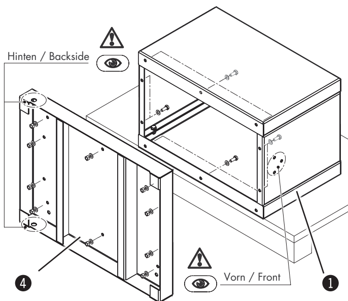
Ábra. 7-2:Szerelés - Gépállvány
