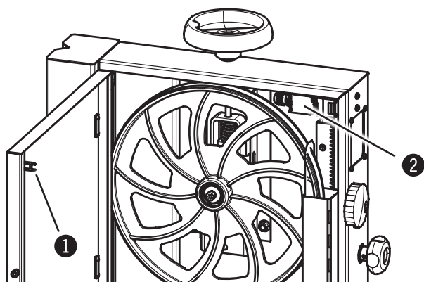
Ábra. 5-3: Reteszelés
