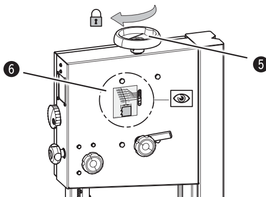
Bild 7-3: Byta bandsågblad
