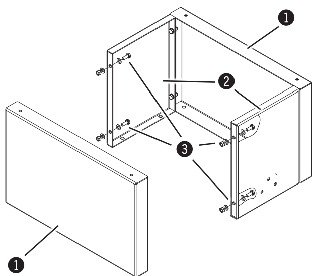
Bild. 7-1: Montering - Maskinstativ
