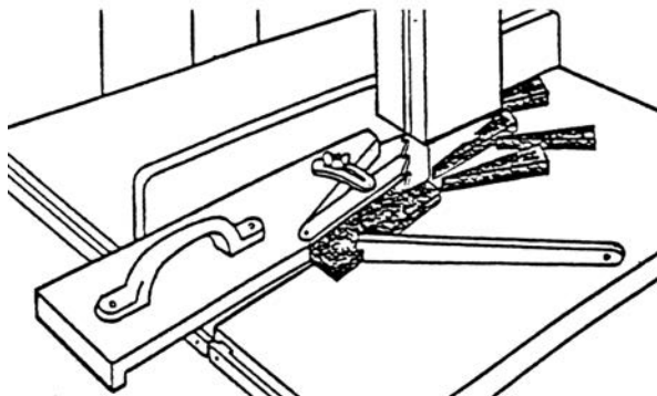
Bild. 8-16: Vinkelsnitt
