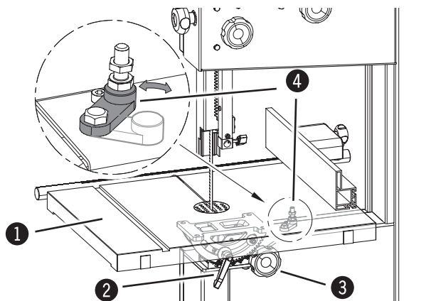
Bild. 8-5: Vinkla
