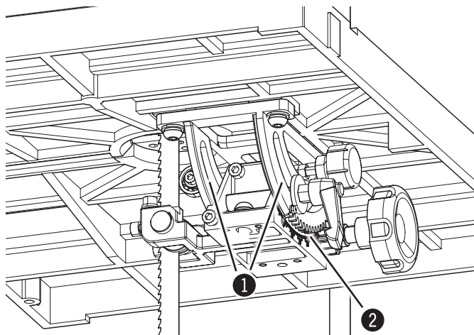
Bild. 9-6: Bordssvängning
