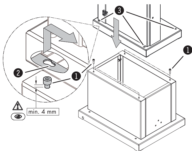
Bild. 7-3: Montering - Bandsågar
