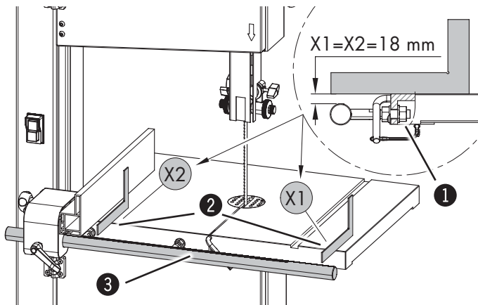
Abb. 7-8: Höheneinstellung - Anschlagführung
