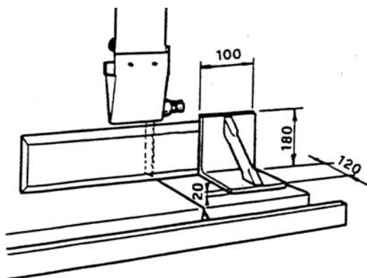
Abb. 8-14: Hilfsanschlag
