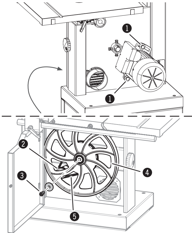
Abb. 9-2: Antriebsriemen austauschen
