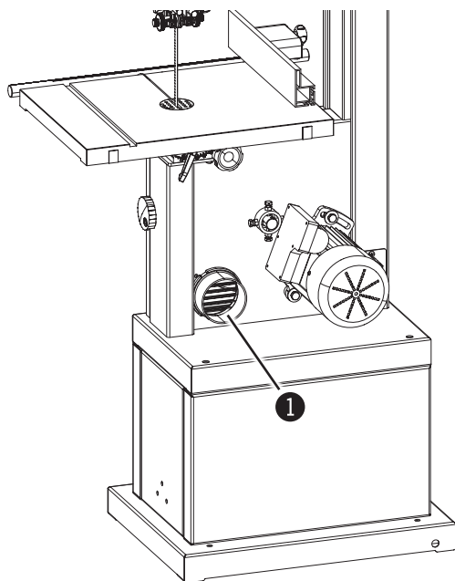
Abb. 4-2: Anschlussstutzen
