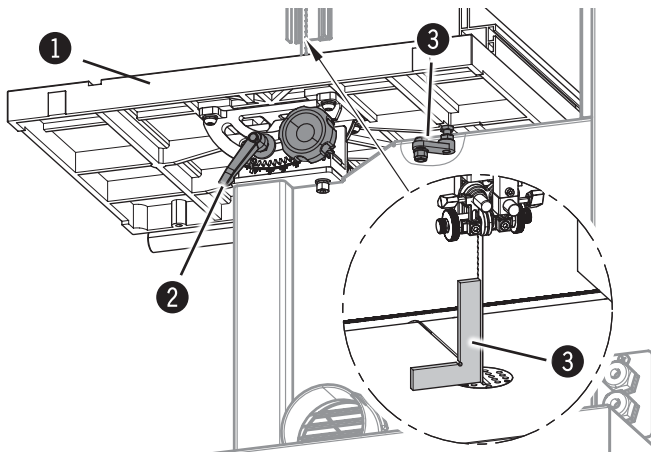
Abb. 7-5: 90° zum Sägebandlauf
