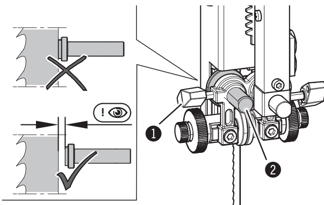
Abb. 8-8: Einstellung der Rückenführung
