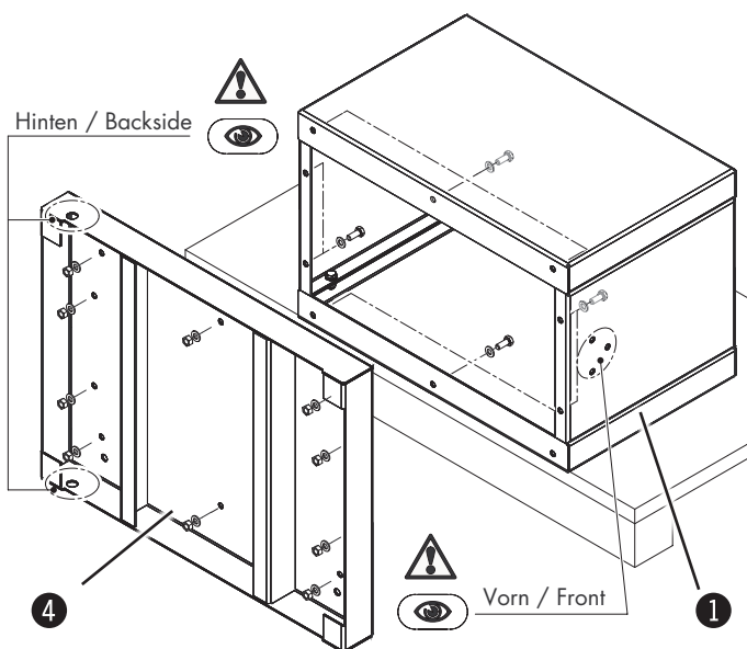
Abb. 7-2: Montage - Maschinengestell
