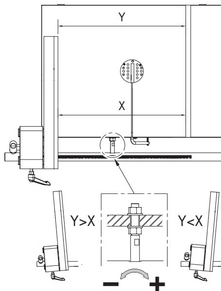
Abb. 9-7: Schnittrichtung und Parallelität
