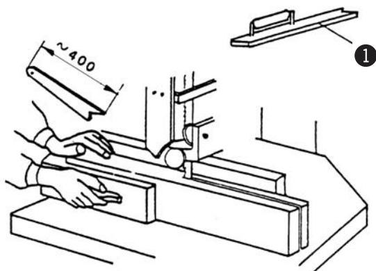
Abb. 8-15: Schiebestock
