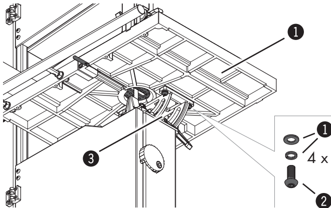
Abb. 7-4: Arbeitstisch
