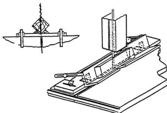
Abb. 8-18: Trennschnitt
