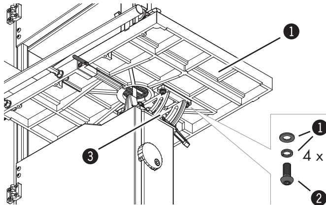
Abb. 7-4: Arbeitstisch
