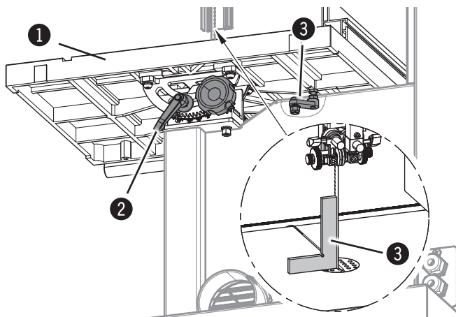
Abb. 7-5: 90° zum Sägebandlauf
