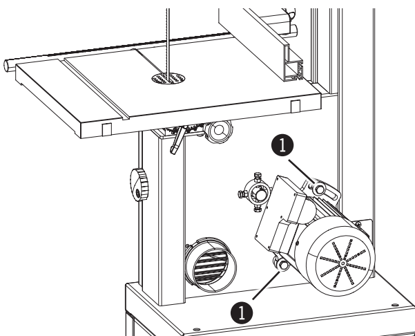
Abb. 9-1: Keilriemen
