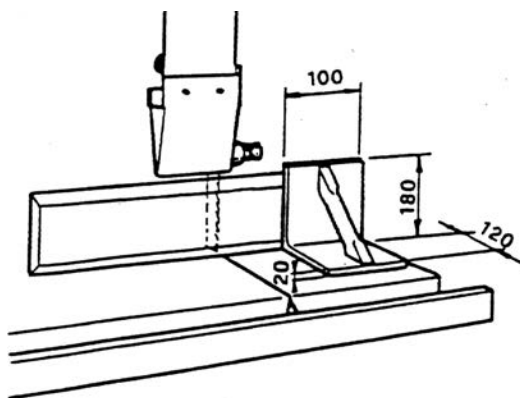
Abb. 8-14: Hilfsanschlag
