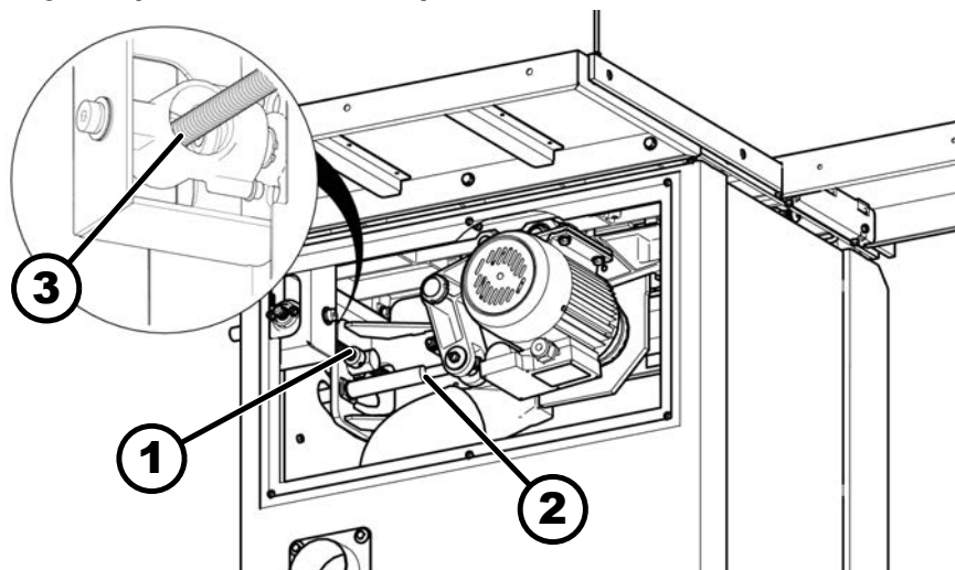
100. ábra: Állítóorsók kenése
