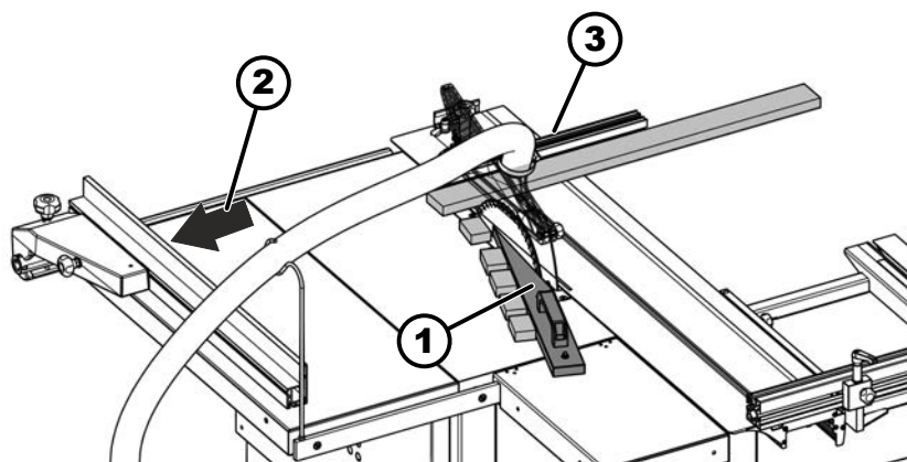
85. ábra: Rövid, keskeny munkadarabok vágása
