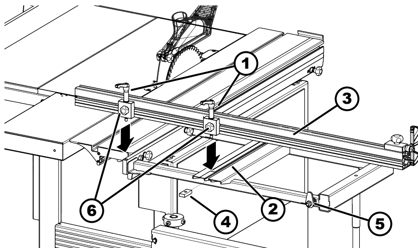
51. ábra: Hosszütköző felszerelése az oldalasztalnál
