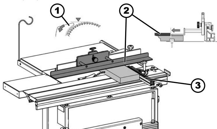
90. ábra: Rejtett vágások hosszütközővel
