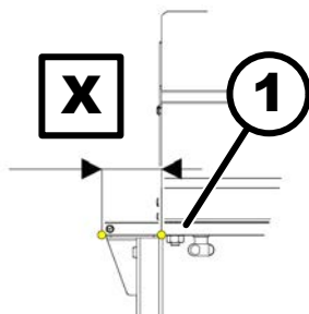
50. ábra: Részlet - Oldalasztal szerelési pozíciója
