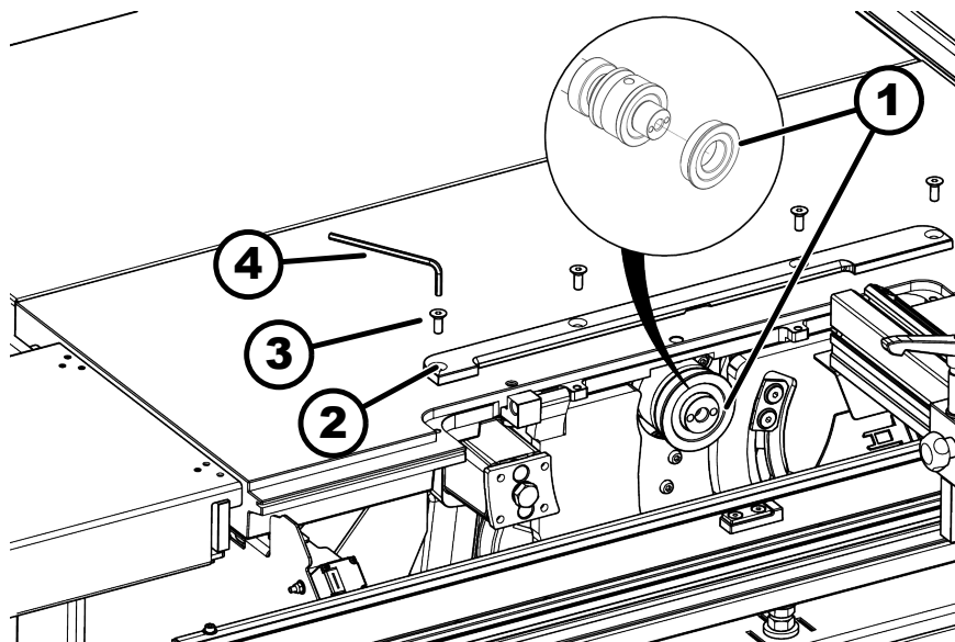
73. ábra: Átalakítás hornyoló szerszámokra
