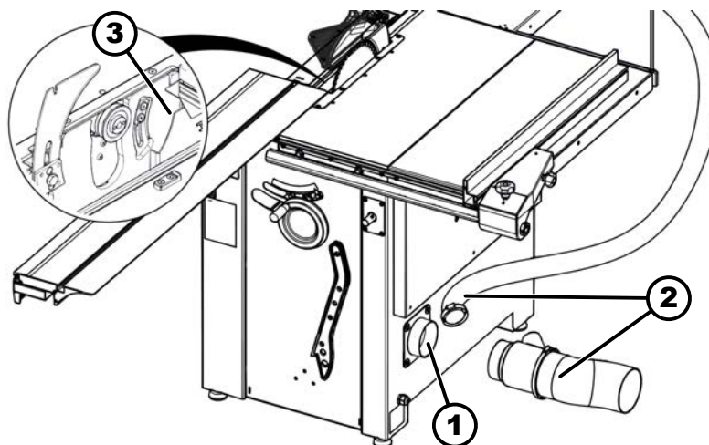
97. ábra: Tisztítsa meg az elszívót.
