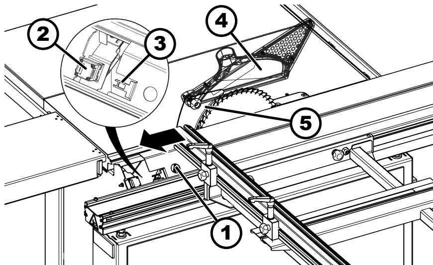
65. ábra: Biztonsági végállaskapcsoló - üzemkész
