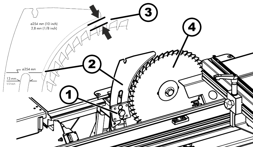
68. ábra: Állítsa be a hasítóéket
