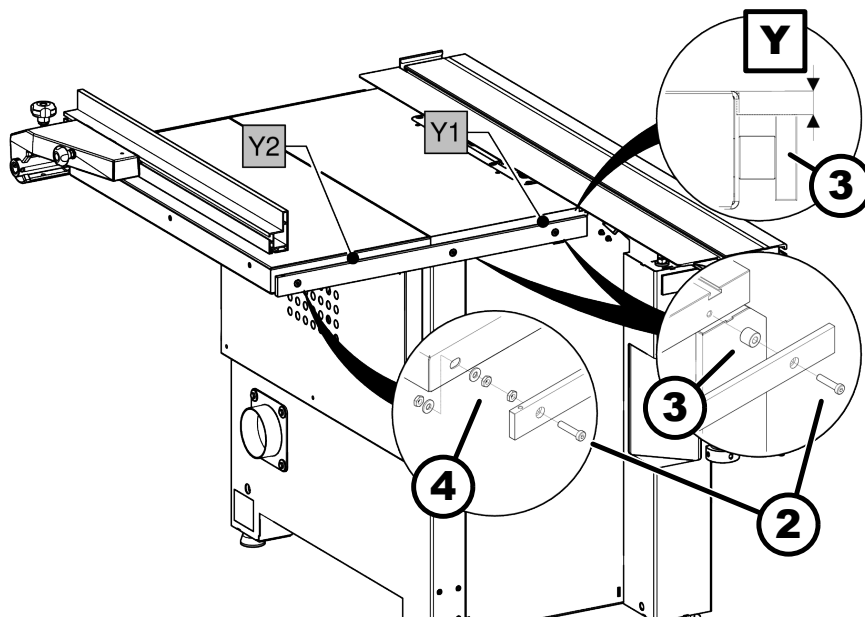
41. ábra: Csatlakoztatórendszer felszerelés
