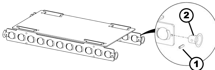
104. ábra: Golyós ketrec - Lehúzó, kaparó
