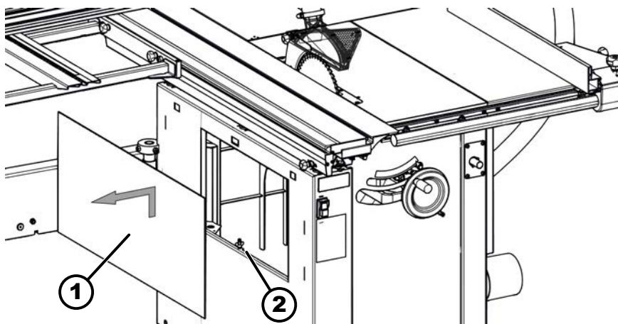
94. ábra: Távolítsa el az elülső borítást
