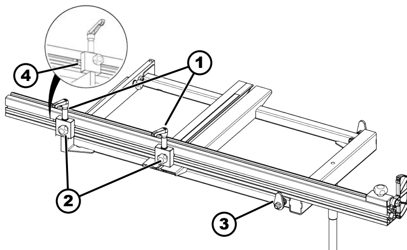
54. ábra: Hosszütköző 0°-os állásban
