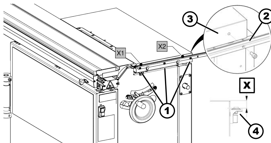
32. ábra: Skálasín felszerelése
