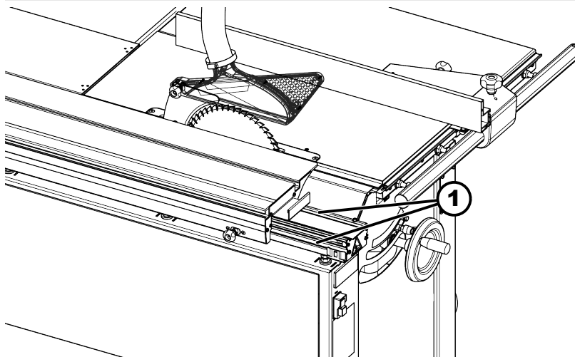
95. ábra: Vezetőfelületek tisztítása
