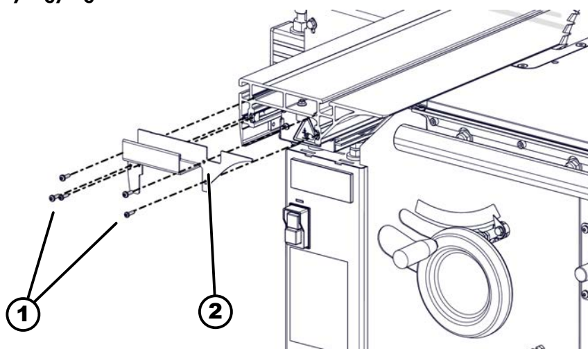
30. ábra: A tolóasztal fogantyúegységének felszerelése
