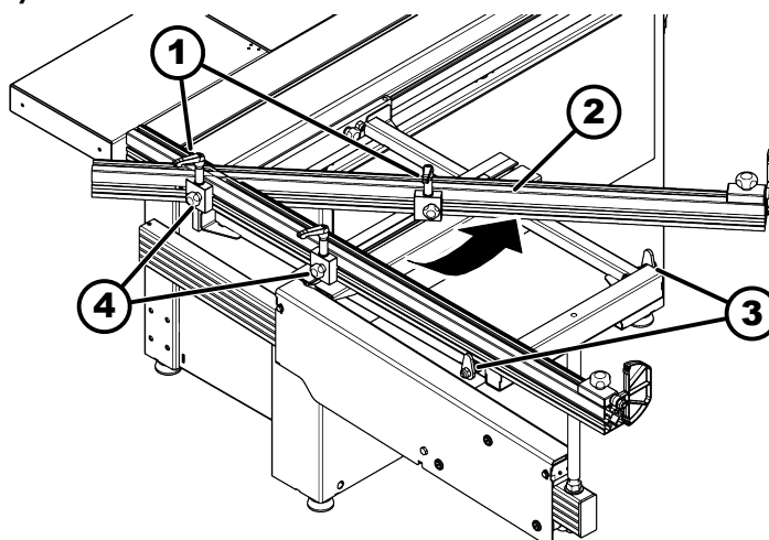
53. ábra: Hosszűtköző elfordítása
