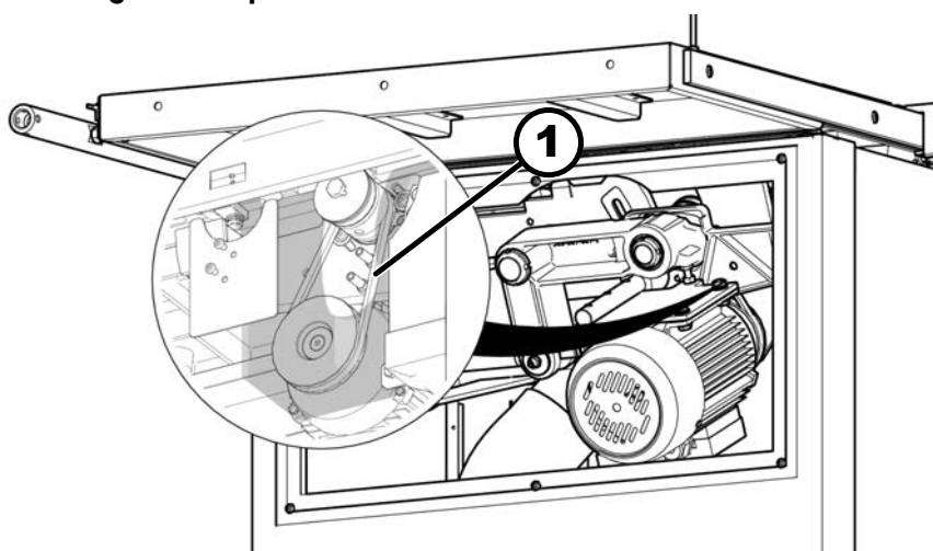
110. ábra: Hajtósíj ellenőrzése
