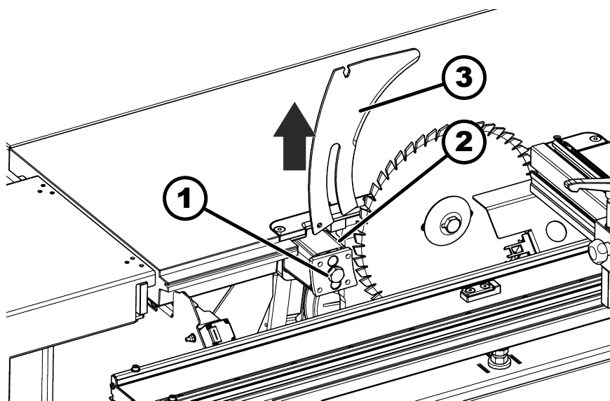
72. ábra: Szerelje ki a hasítóéket
