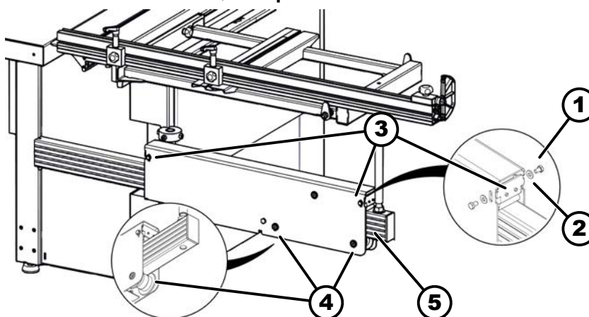
96. ábra: Kefesor, oldalasztal-konzolja
