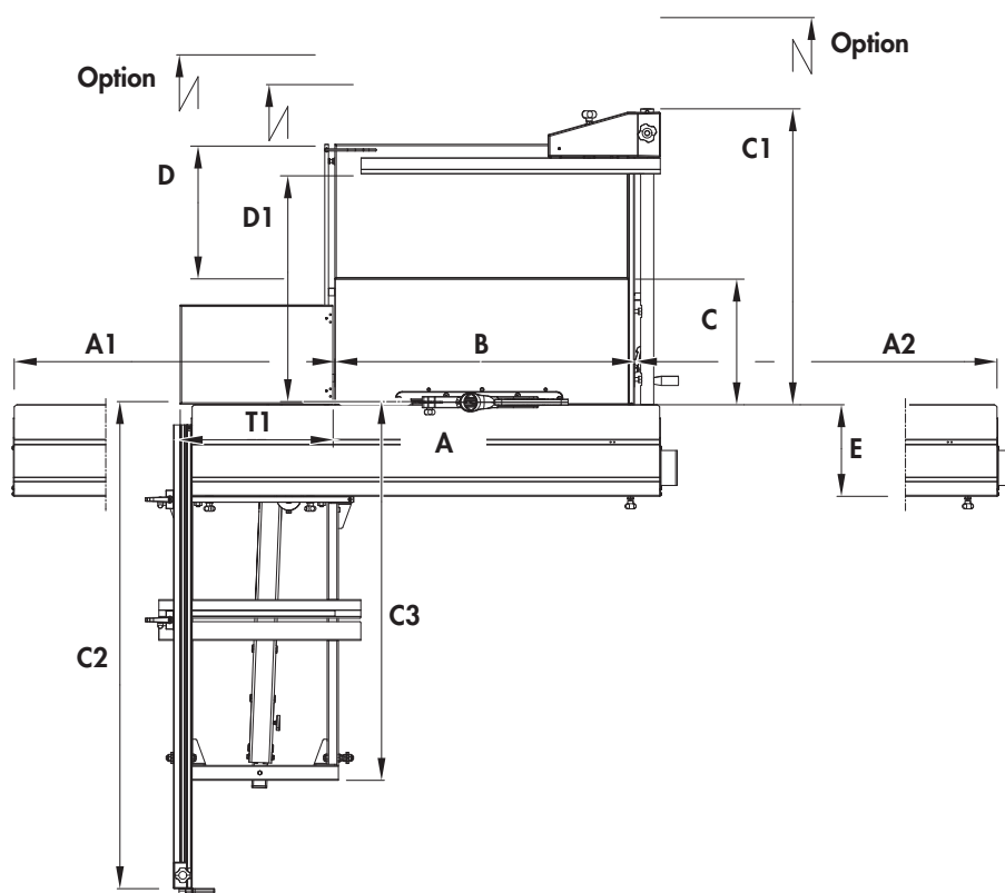
2. ábra: Méretek K2S - vágási szélességek
