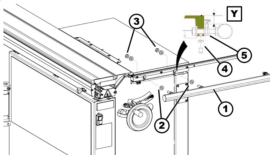
33. ábra: Ütközőtengely felszerelése
