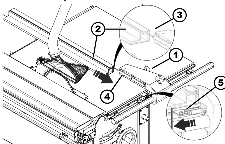
58. ábra: Lapos vonalzó beszerelése
