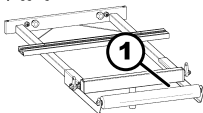
14. ábra: Oldalasztal meghosszabbítása
