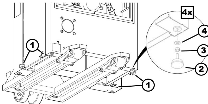
21. ábra: Előkészítés az emelőkocsi szállításra
