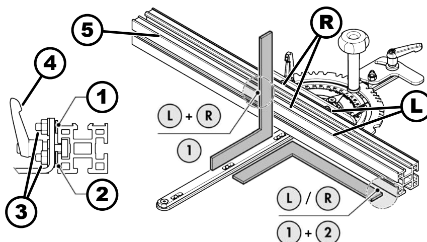
116. ábra: Hosszűtköző - szög helyesbítése
