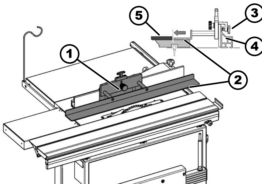
61. ábra: „Fűrész boy” segédütköző felszerelése
