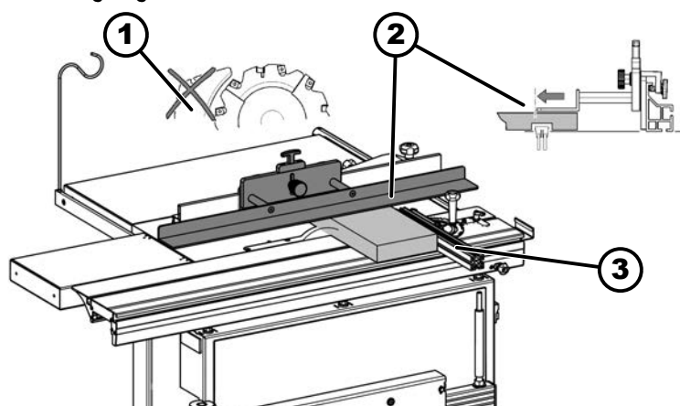
92. ábra: Hornyoló munkák hosszütközővel
