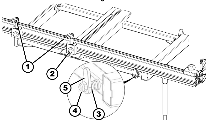
118. ábra: Hosszütköző 0°-os szög helyesbítése
