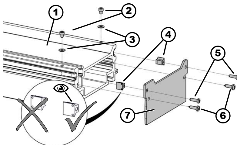
107. ábra: Alappálya-burkolat
