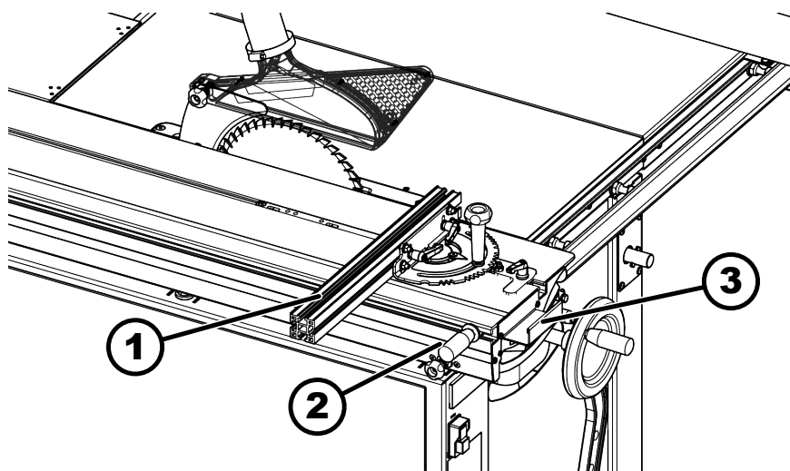
80. ábra: Tolóasztal eltolása
