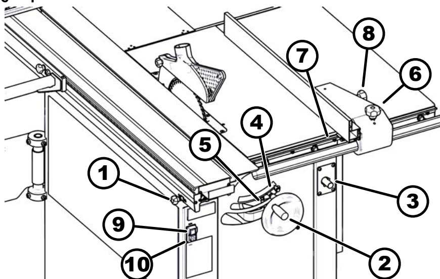
16. ábra: A vezérlők áttekintése
