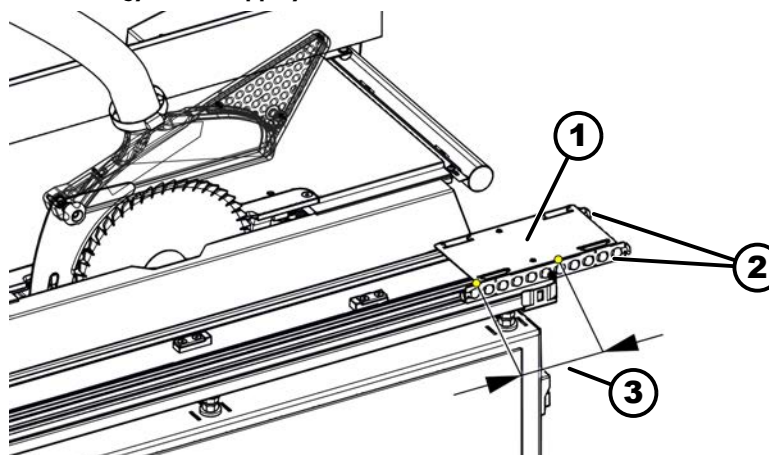
105. ábra: Alappálya golyós ketrecel
