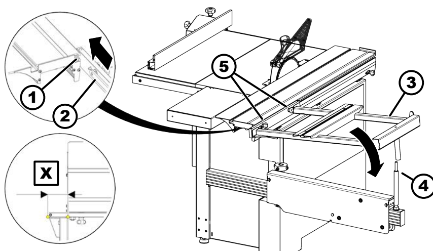
49. ábra: A Oldalasztal felszerelése
