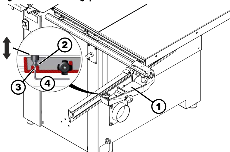
113. ábra: Párhuzamüt-köző magasságának utánállítása
