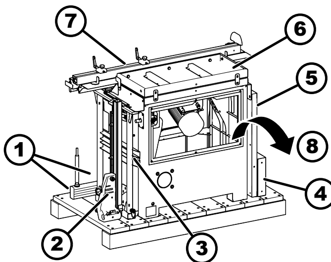
20. ábra: Felszerelhető alkatrészek eltávolítása
