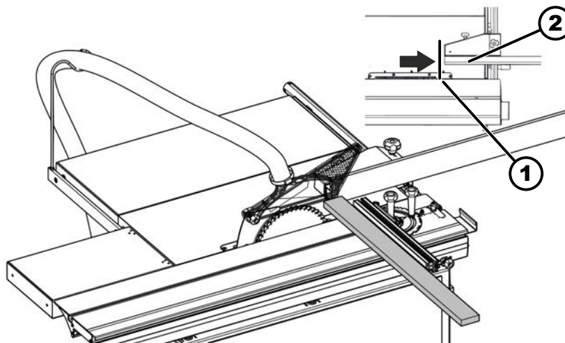
86. ábra: Darabolás a párhuzamütközőnél
