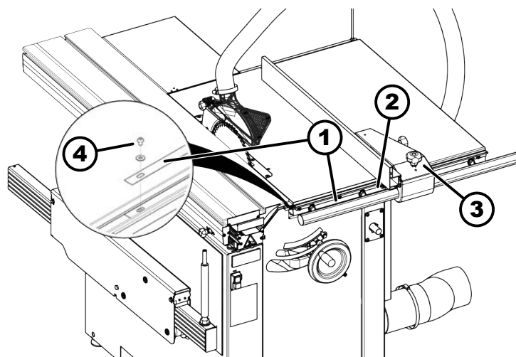
57. ábra: A párhuzaműtköző eltolása
