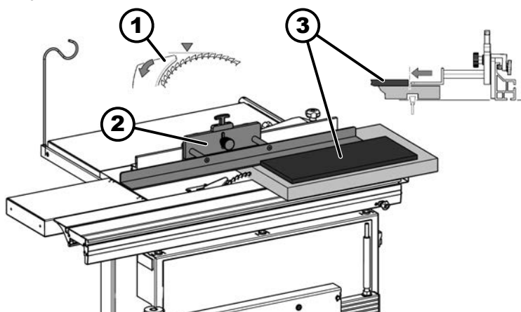
89. ábra: Rejtett vágások sablonnal
