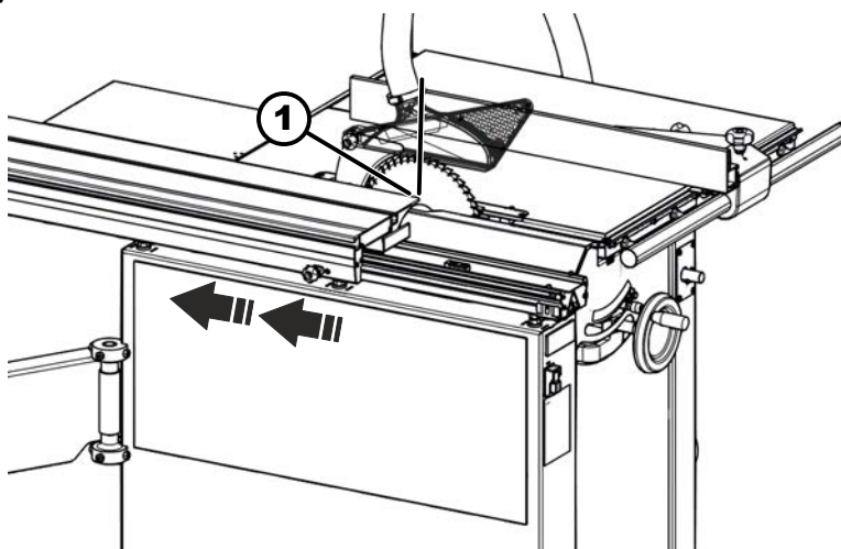
109. ábra: A tolóasztal golyókosarának beállítása
