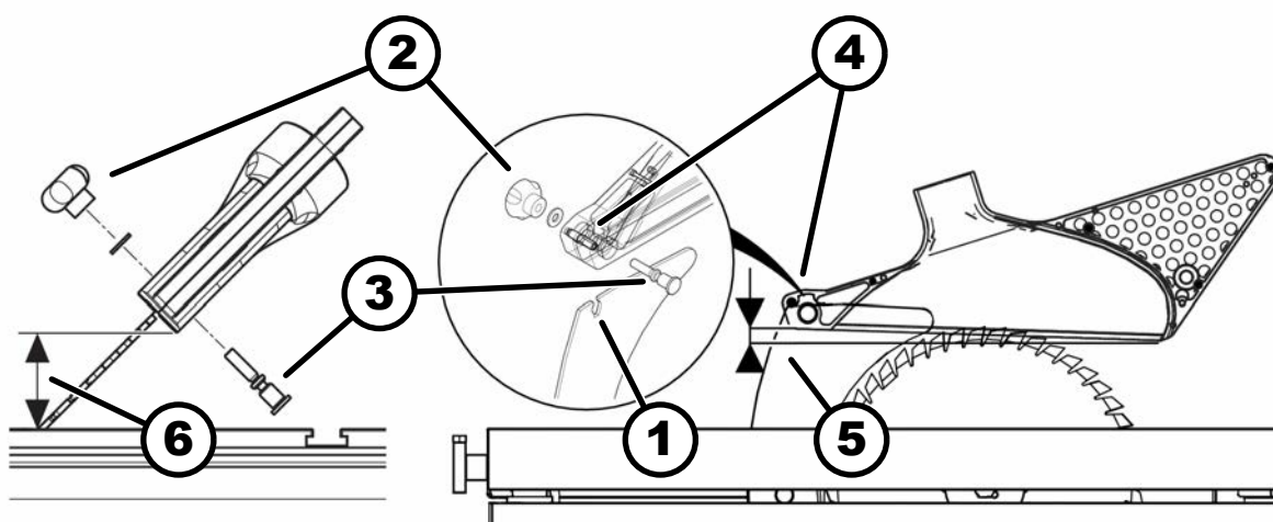
78. ábra: A körfűrészvédő fedél beállítása
