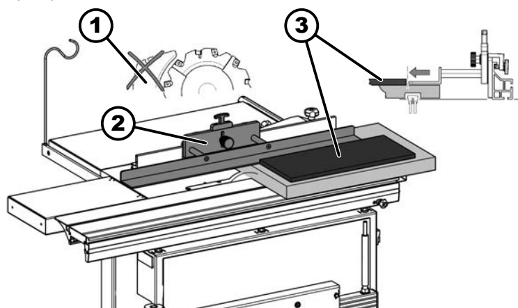
91. ábra: Hornyoló munkák sablonnal
