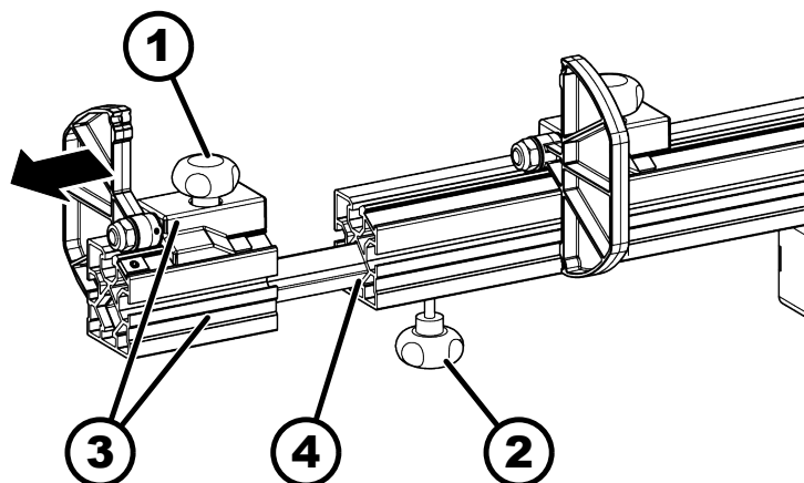
56. ábra: Hosszütköző-hosszabbító
