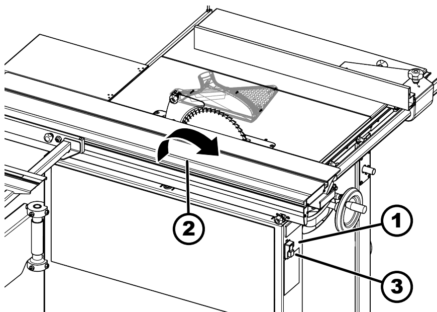
45. ábra: Motor fűrésiránya
