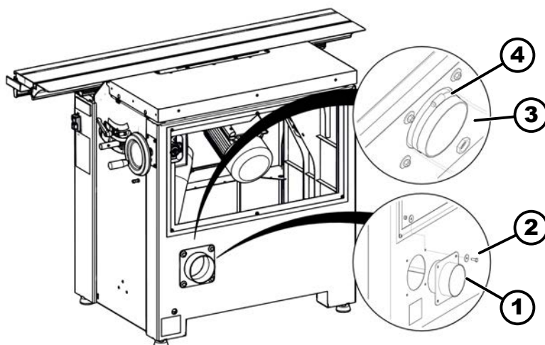
28. ábra: Az elszívócsonk felszerelése
