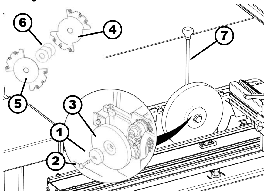
74. ábra: Hornyoló szerszám beszerelése
