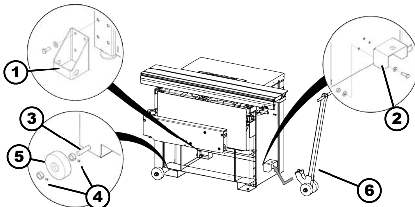
24. ábra: Kirakodás mozgatóberendezéssel
