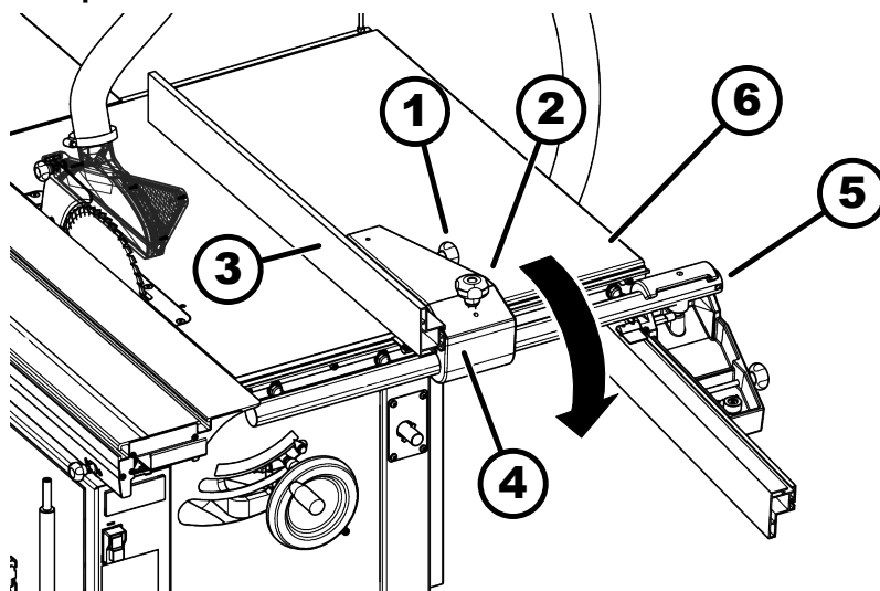
60. ábra: Párhuzamütköző lehajtása
