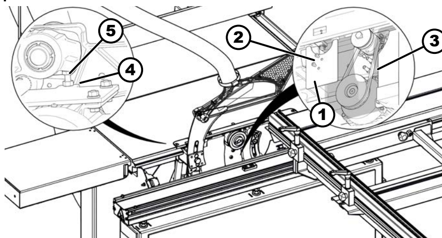
111. ábra: A hajtósíj cseréje
