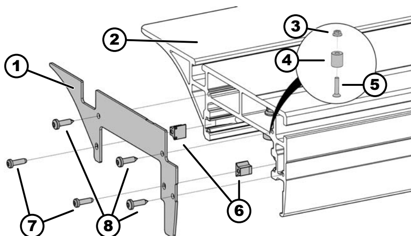
108. ábra: A tolóasztal eltávolítása - fedél
