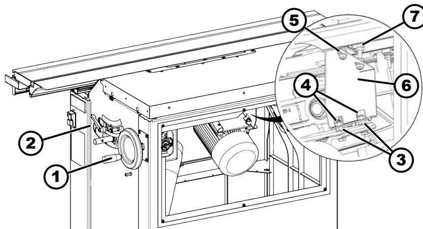
27. ábra: A gépegység szállítási biztosításának eltávolítása
