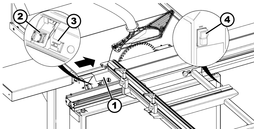
98. ábra: Biztonsági kapcsoló tolófedele
