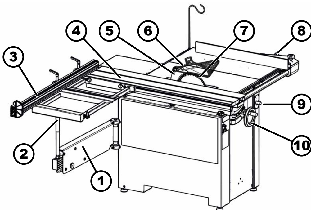
5. ábra: Elülső oldal áttekintése
