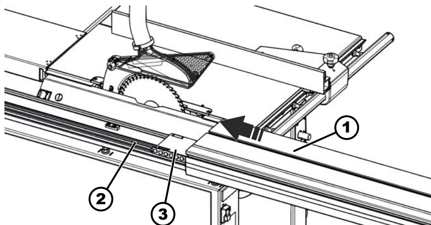
106. ábra: Tolóasztal felszerelése
