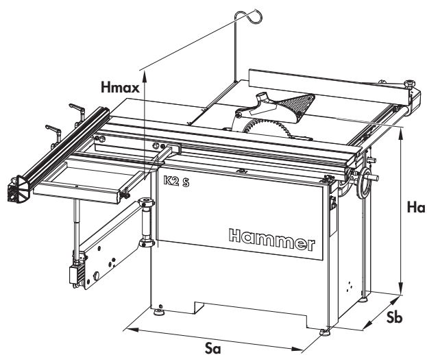
1. ábra: Méretek K2S - alapgép
