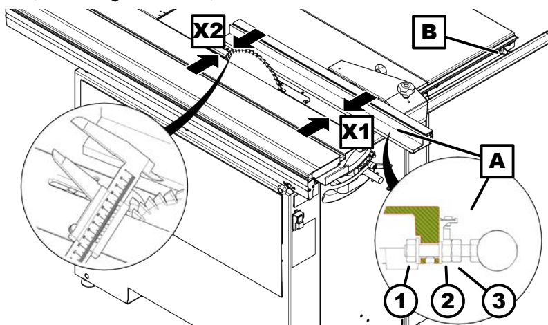
115. ábra: Szabad vágás beállítása
