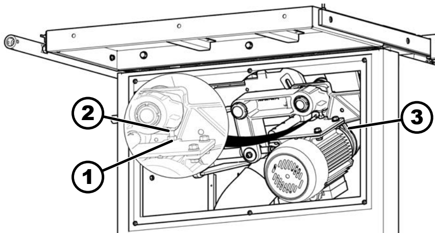
112. ábra: A hajtósíj utánfeszítése
