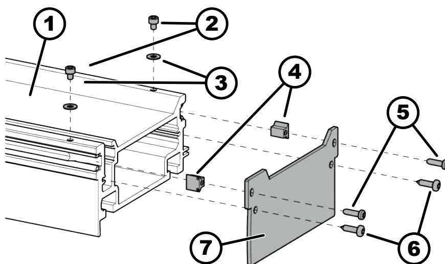
101. ábra: Alappálya-burkolat
