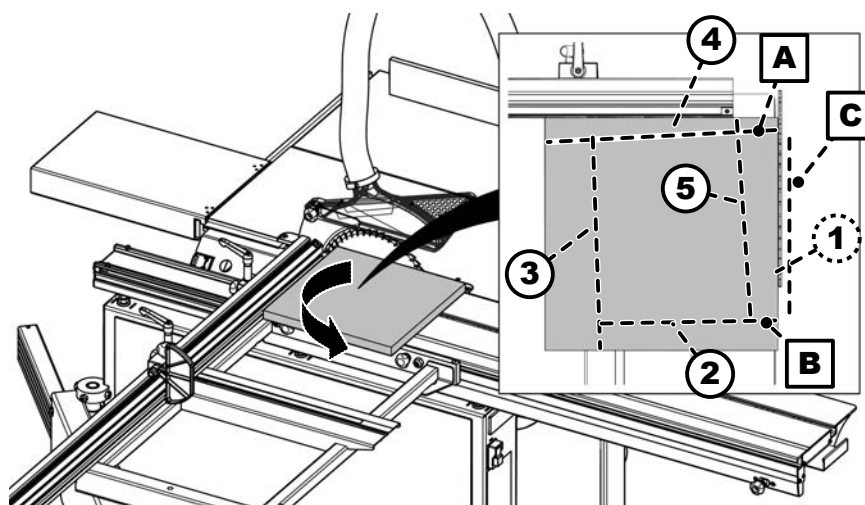
119. ábra: Próbavágás - 5 oldalas vágás
