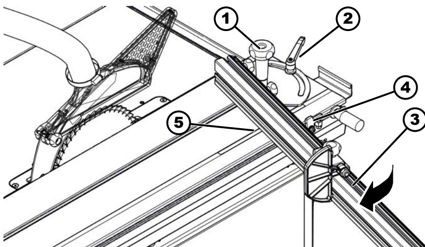
48. ábra: Hosszütköző elfordítása
