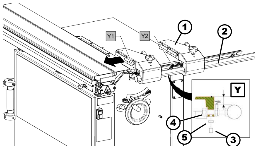
34. ábra: Ütközőtengely - ellenőrzés
