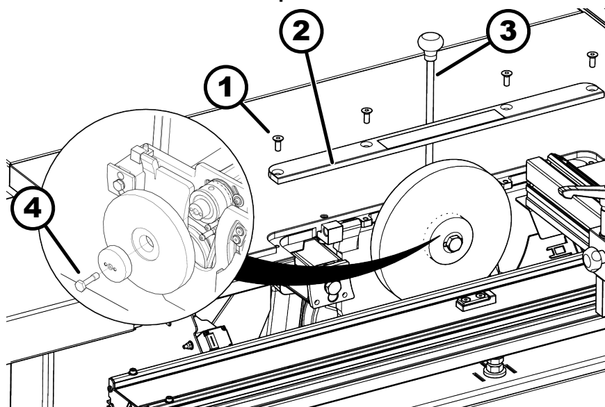
76. ábra: Hornyoló szerszám kiszerelése
