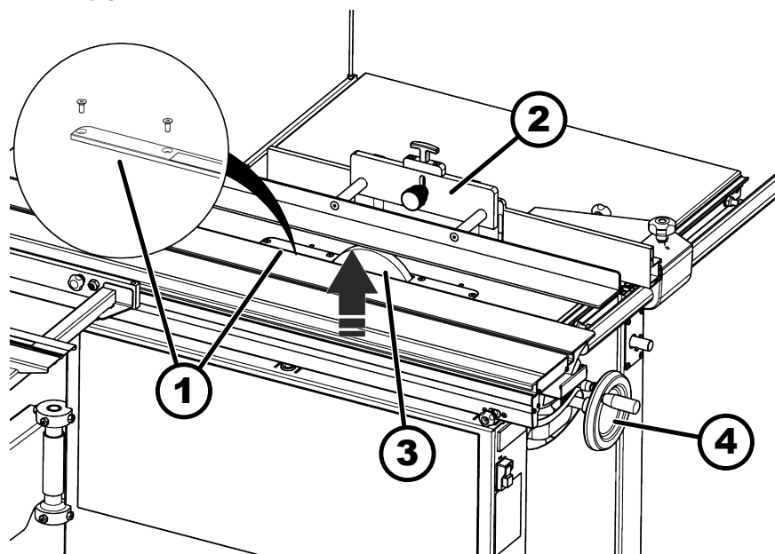
75. ábra: Betétlap hornyoló szerszámok beépítéséhez
