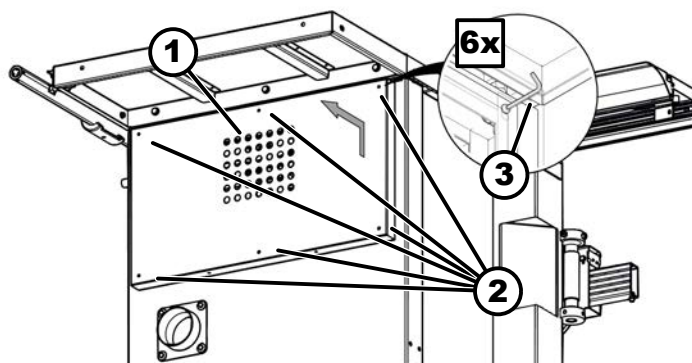
93. ábra: Távolítsa el a hátsó burkolatot
