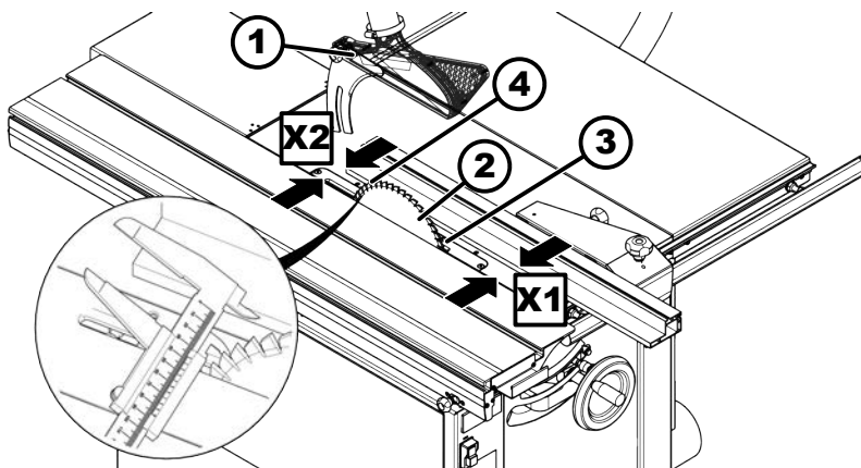
114. ábra: Szabad vágás előkészítése
