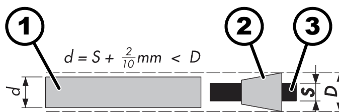
70. ábra: Fűrészlaphoz illő feszítőék
