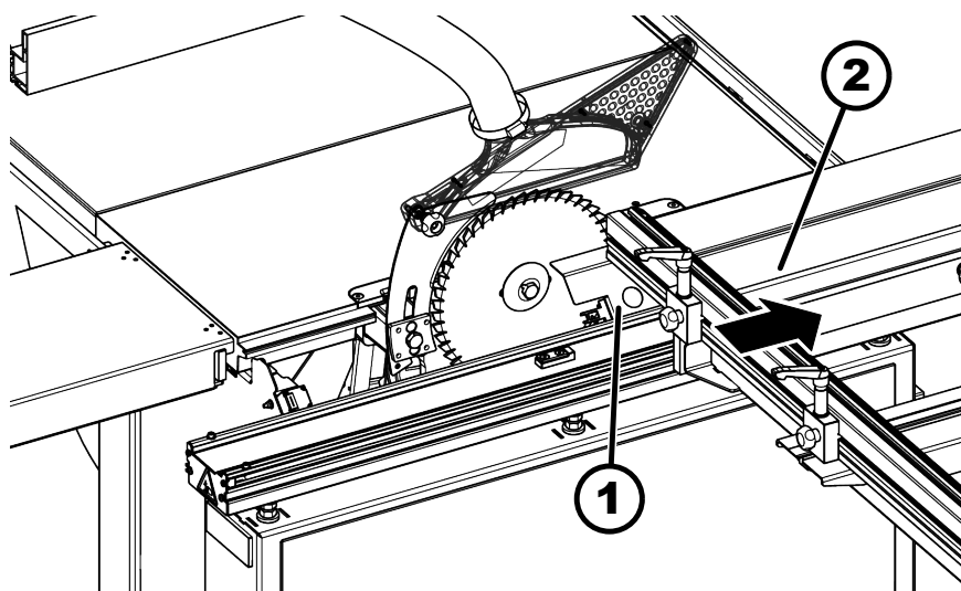
64. ábra: Előkészület szerszámcserehez
