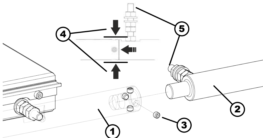
37. ábra: 1220-as hosszabbítótengely felszerelése
