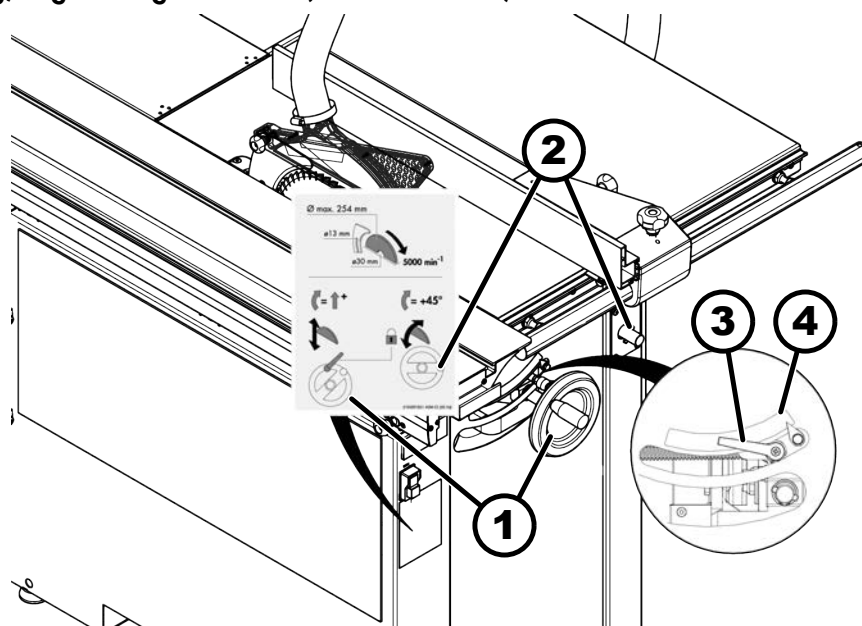
62. ábra: Vágásmagasság/vágási szög beállítása
