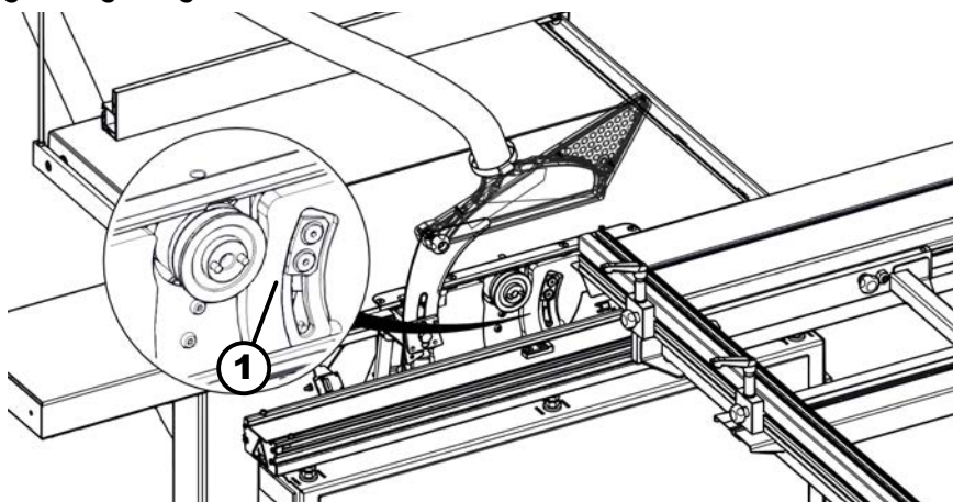
99. ábra: Magassági megvezetés kenése
