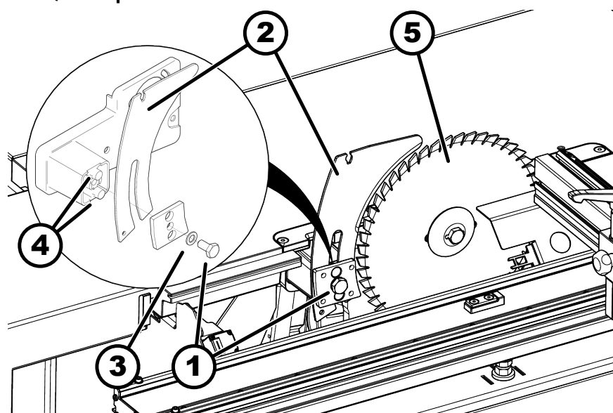
69. ábra: Feszítőék beszerelése
