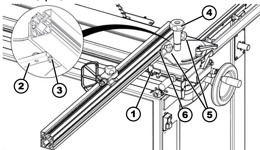
47. ábra: Hosszűtköző a tolóasztalon
