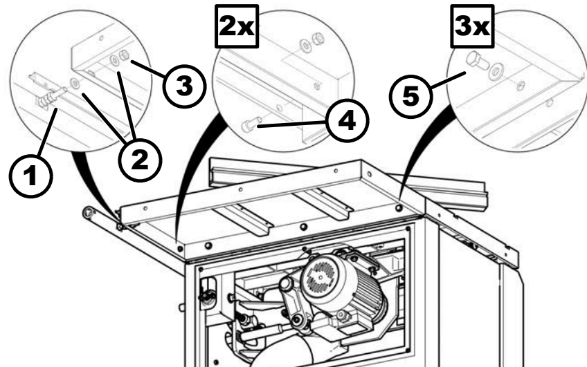
Afb. 26: Zaagverbreding monteren - Variant 610
