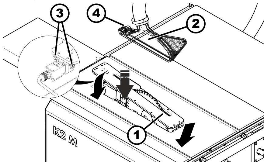
Afb. 45: Bedrijfsklaarheid - Cirkelzaag werken
