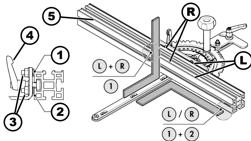
Afb. 79: Afkortaanslag - hoek corrigeren
