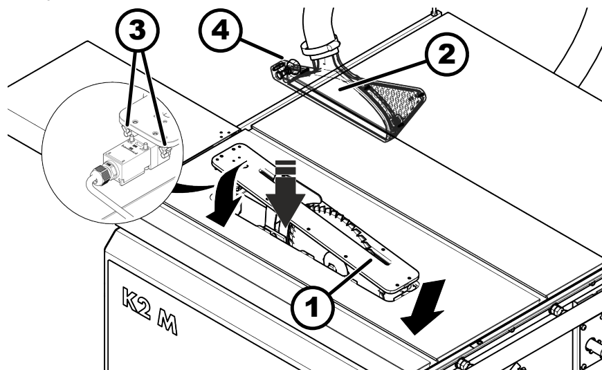
Afb. 57: Bedrijfsklaarheid - Cirkelzaag werken
