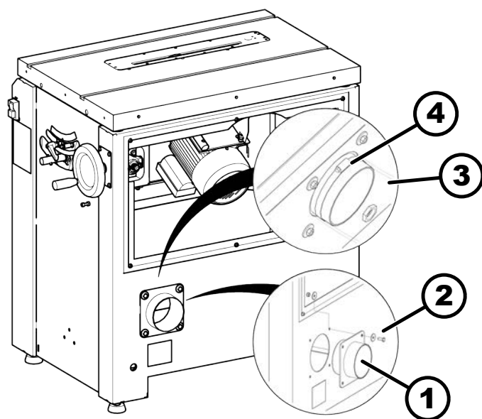
Afb. 22: Afzuigmonden monteren
