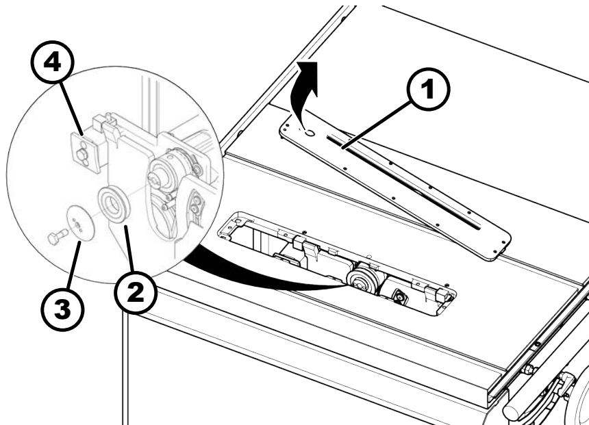
Afb. 53: Achterste flens/spouwmeshouder/inlegplank
