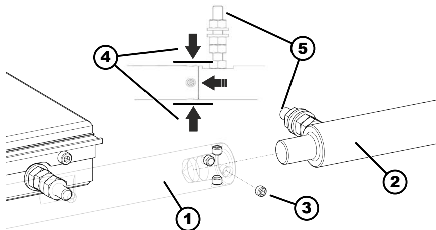
Afb. 28: Verlengingsas 1220 monteren
