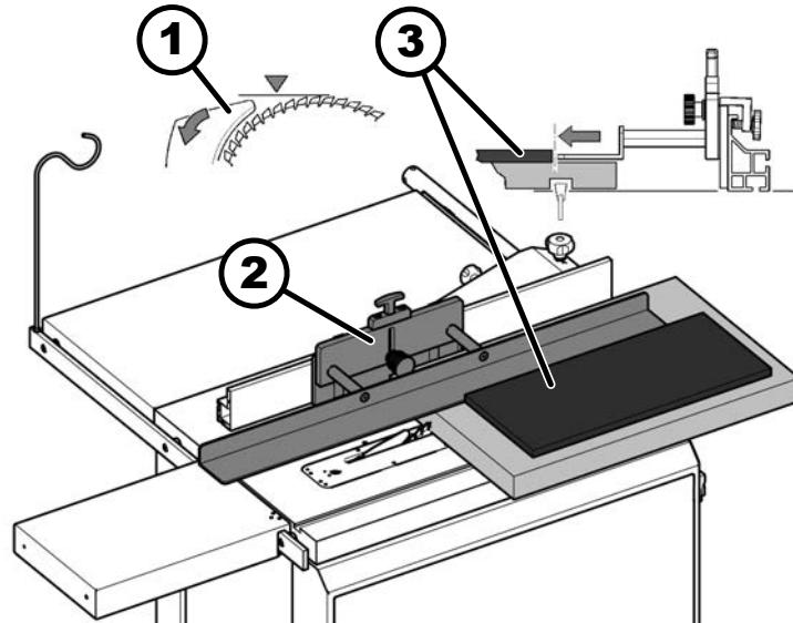
Afb. 65: Verdekete snedes met sjabloon
