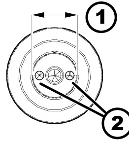
Afb. 43: Antiverdraaiingsinrichting zaagas
