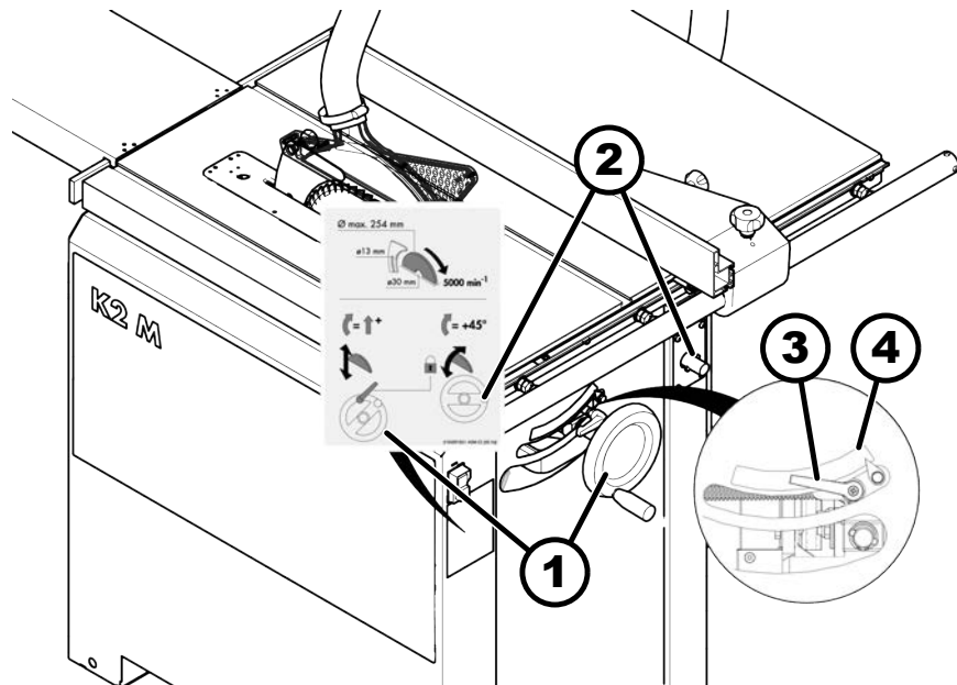
Afb. 42: Zaaghoogte/zaaghoek instellen
