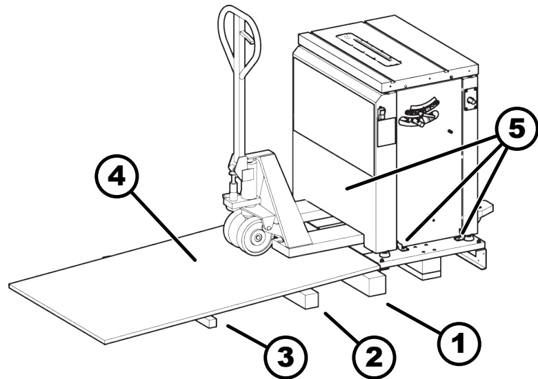
Afb. 16: Afladen met palletwagen
