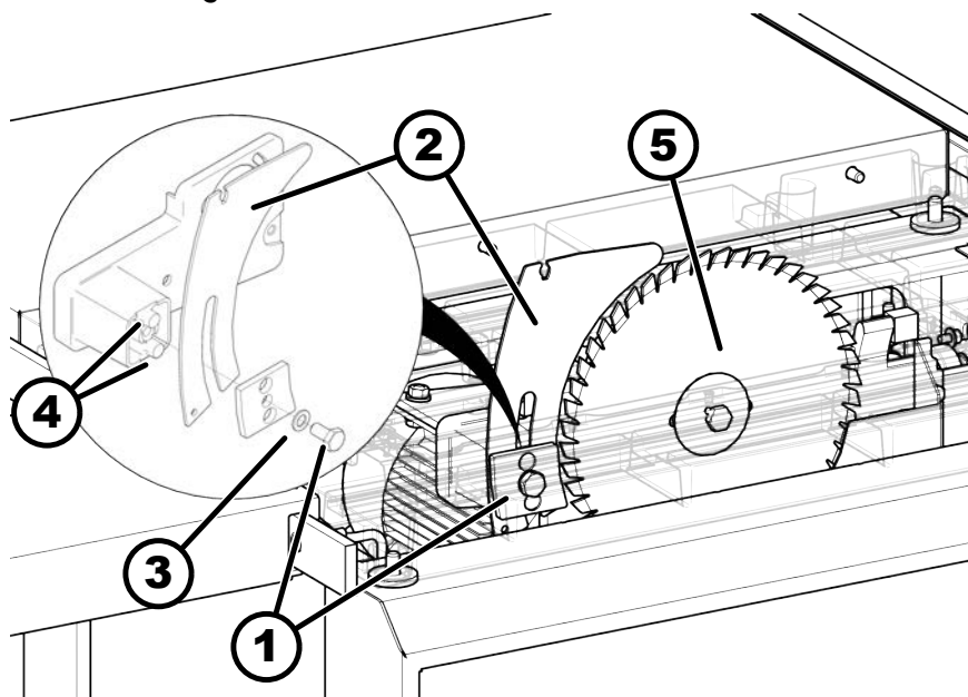
Afb. 49: Spouwmes monteren
