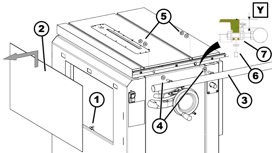
Afb. 24: Aanslagas monteren
