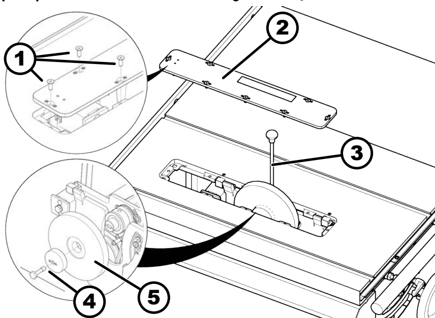
Afb. 56: Groefgereedschap demonteren
