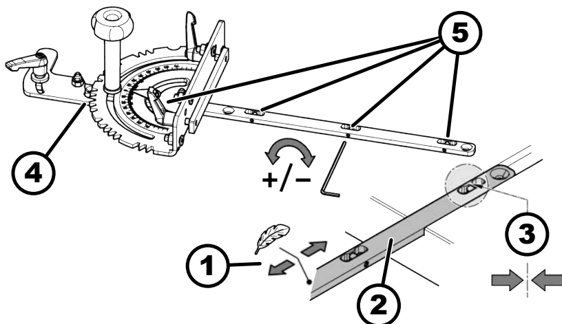
Afb. 81: Afkortaanslag - Railbreedte instellen
