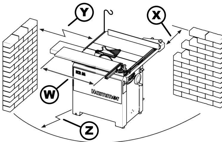
Afb. 19: Benodigde ruimte K2 M
