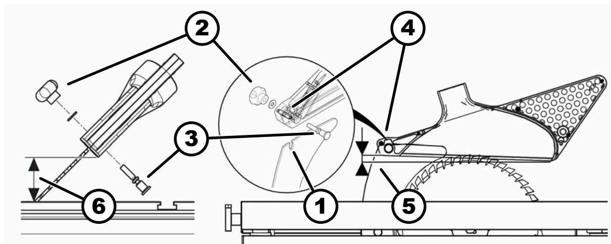
Afb. 58: Beschermkap cirkelzaag instellen
