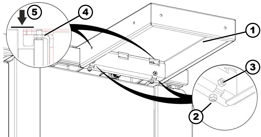
Afb. 33: Tafelverlenging instellen
