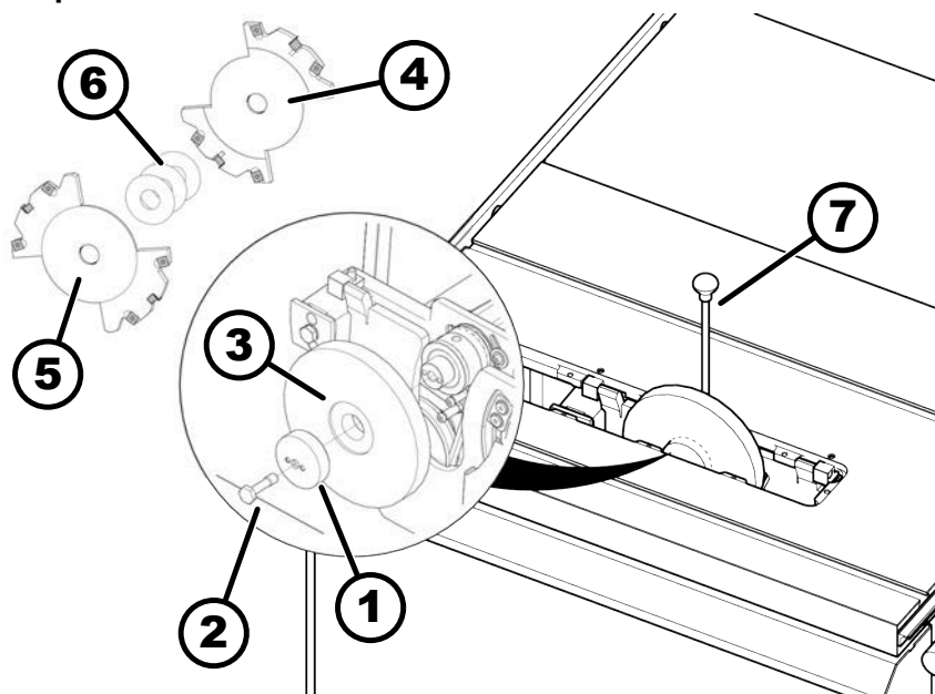
Afb. 54: Groefgereedschap monteren
