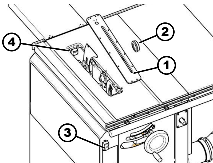
Afb. 70: Veiligheidsschakelaar Insteekkaart
