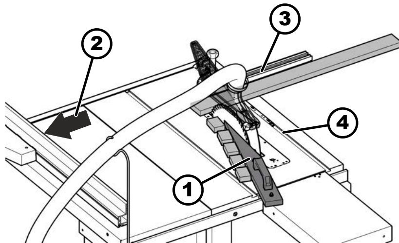
Afb. 63: Korte, smalle werkstukken zagen
