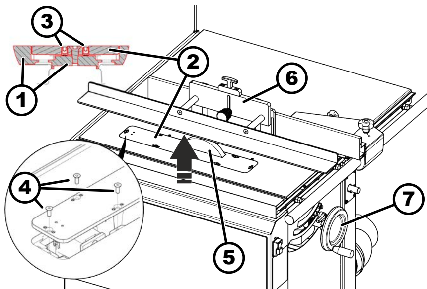
Afb. 55: Inlegplank voor groefgereedschap monteren
