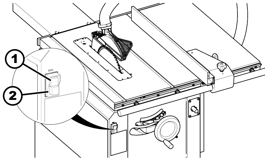
Afb. 59: In- / Uitschakelen
