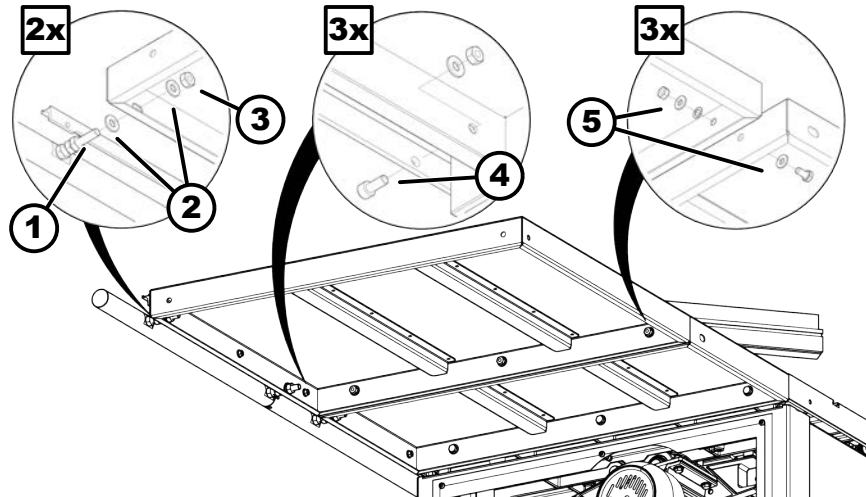
Afb. 29: Zaagverbreding monteren - Variant 1220
