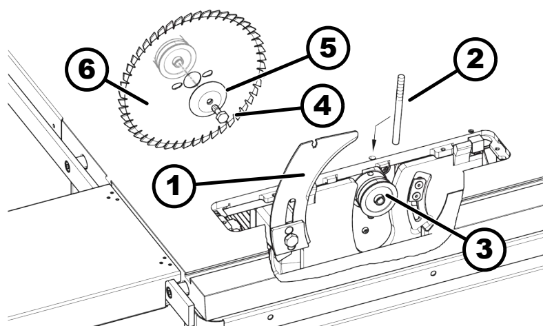
Afb. 47: Zaagblad vervangen
