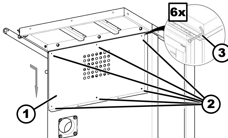
Afb. 27: Afdichtdeksel monteren
