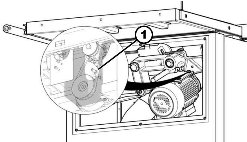
Afb. 73: Aandrijfriem controleren
