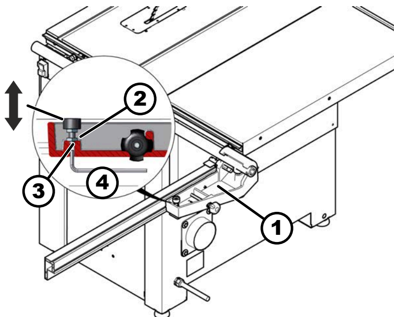
Afb. 76: Hoogte parallelaanslag bijstellen
