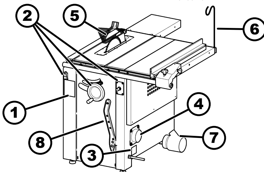
Afb. 5: Overzicht Achterzijde
