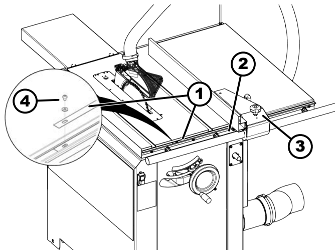
Afb. 37: Parallelaanslag verschuiven
