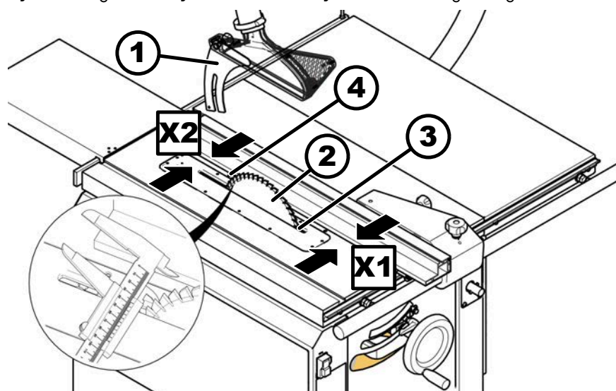
Afb. 77: Vrije snede voorbereiden
