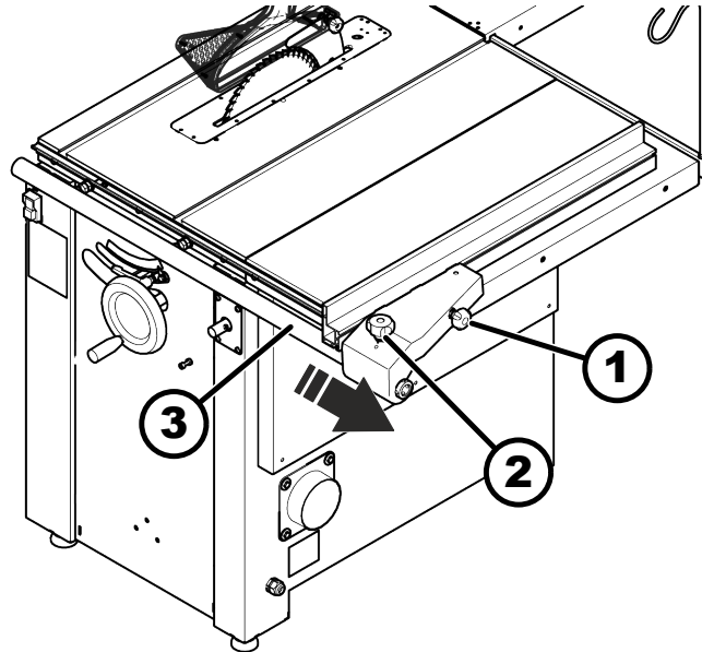
Afb. 39: Parallelaanslag verwijderen
