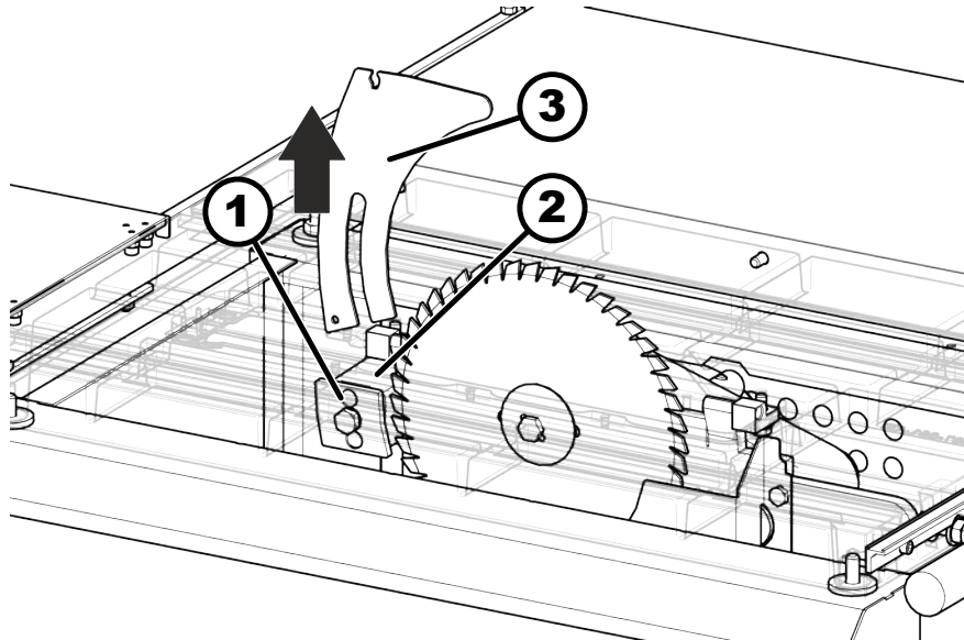
Afb. 52: Spouwmes demonteren
