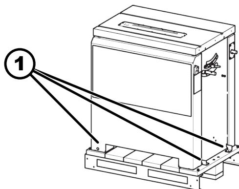
Afb. 13: Transporthoek verwijderen
