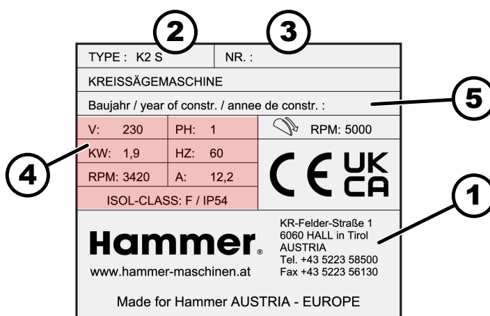
Afb. 8: Typeplaatje
