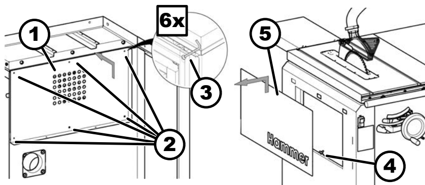
Afb. 69: Afdekking verwijderen
