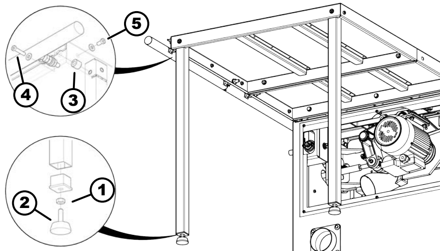
Afb. 30: De steunvoet aanbrengen
