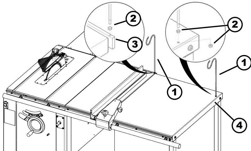
Afb. 34: Borgveer afzuigbuis monteren
