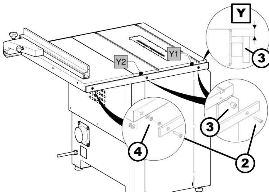
Afb. 32: Koppelsysteem monteren
