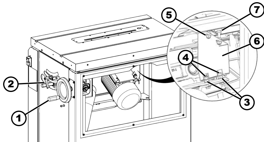
Afb. 21: Transportbeveiliging aggregaat verwijderen
