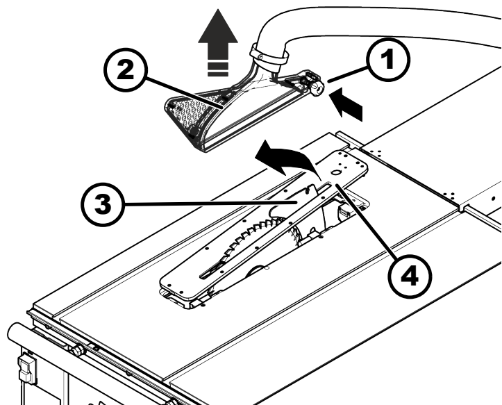
Afb. 44: Voorbereiden voor gereedschapswissel
