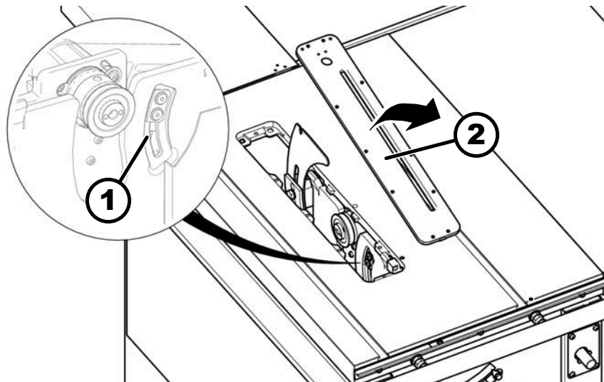
Afb. 71: Hoogtegeleiding smeren
