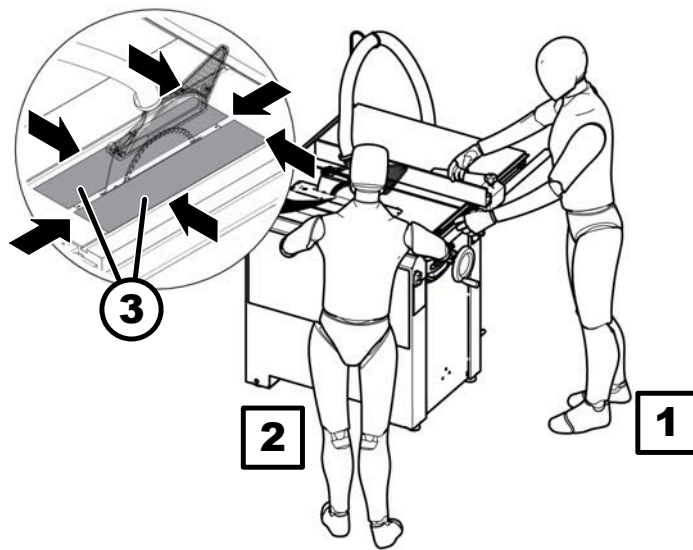
Afb. 60: Werkposities
