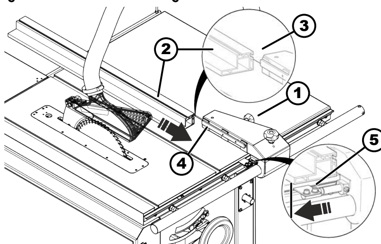
Afb. 38: Liniaal vlak monteren
