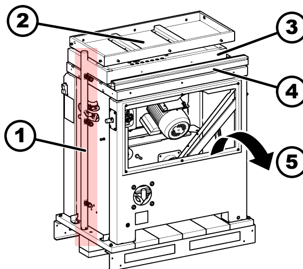
Afb. 14: Aanbouwdelen verwijderen
