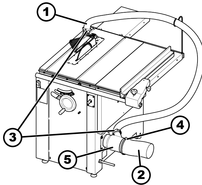
Afb. 35: Afzuigaansluiting
