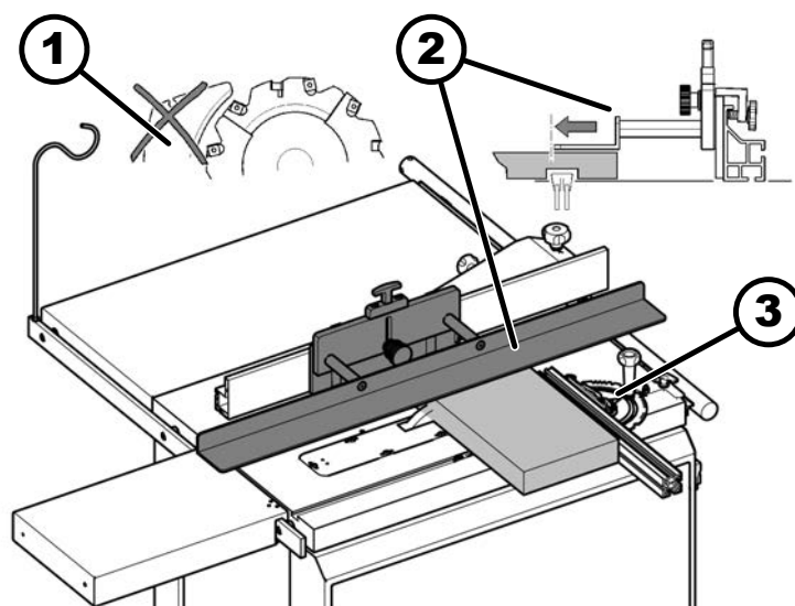
Afb. 68: Groefbewerkingen met afkortaanslag
