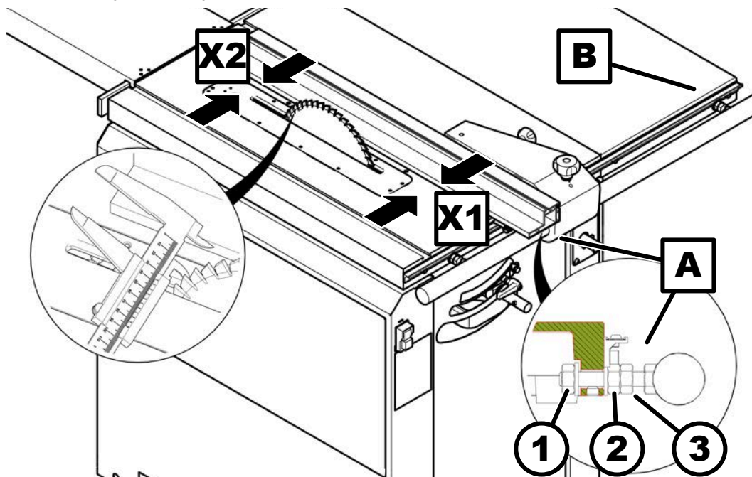
Afb. 78: Vrije snede Instellen
