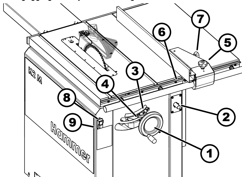
Afb. 10: Overzicht bedieningselementen
