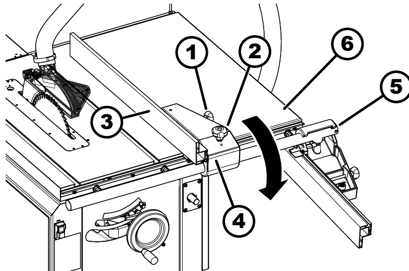
Afb. 40: Parallelaanslag wegzwenken
