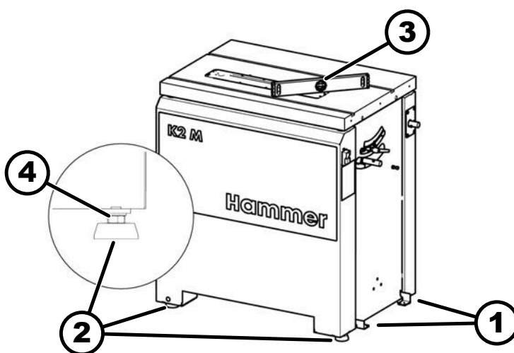
Afb. 20: Machine uitlijnen
