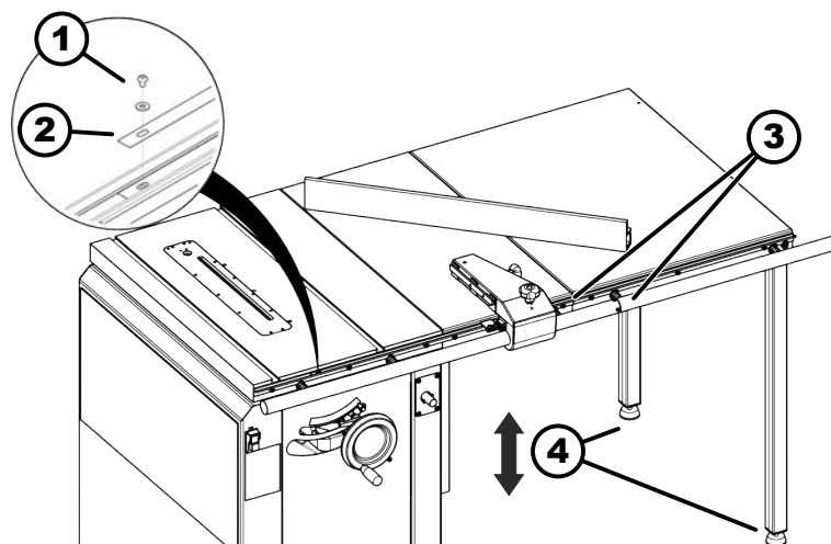
Afb. 31: Zaagverbreding 1220
