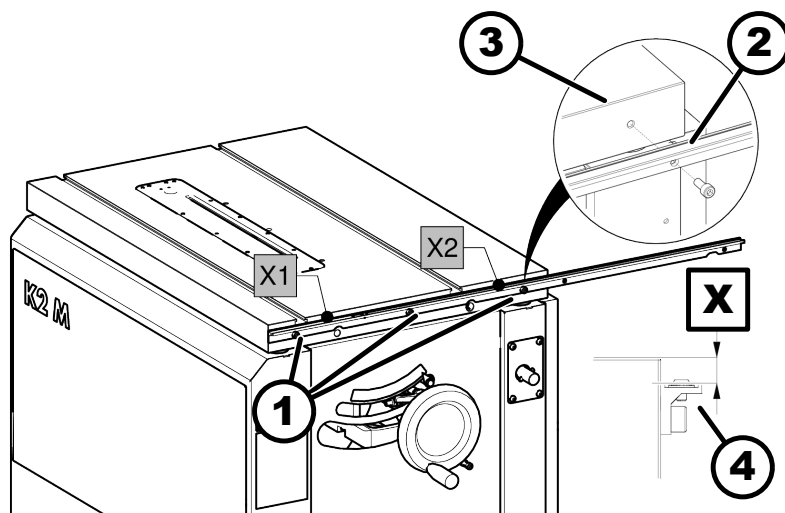
Afb. 23: Maatverdelingsrail monteren
