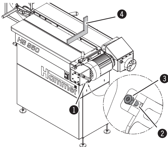
Fig. 11-3: Ajuste del ángulo - 0°
