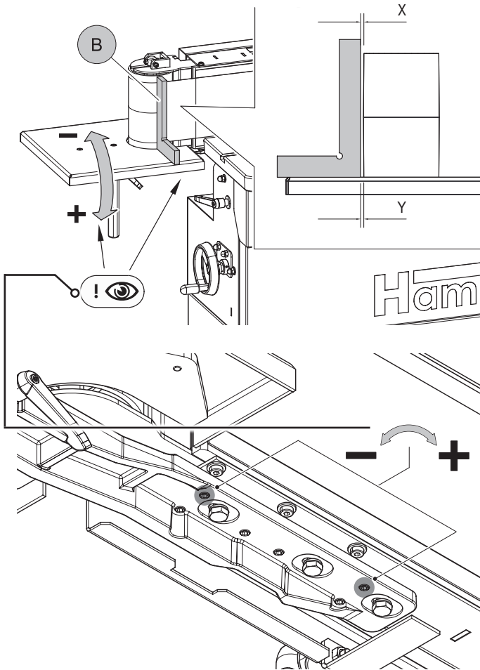
Fig. 7-13: Ajuste - Ángulo B
