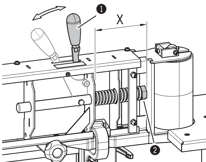
Fig. 11-1: Ajustar la tensión del muelle
