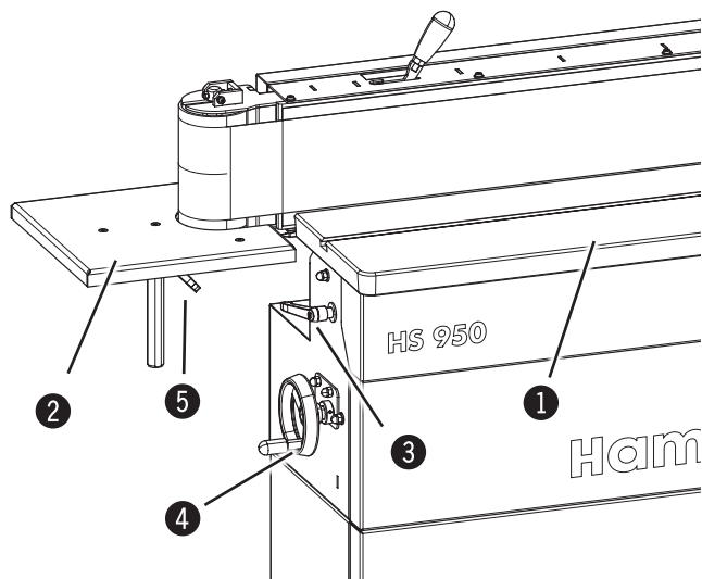
Fig. 8-3: Ajuste de la altura de la mesa de trabajo
