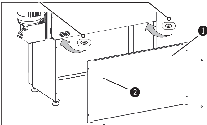
Fig. 10-1: Preparación - Lubricar el ajuste de altura
