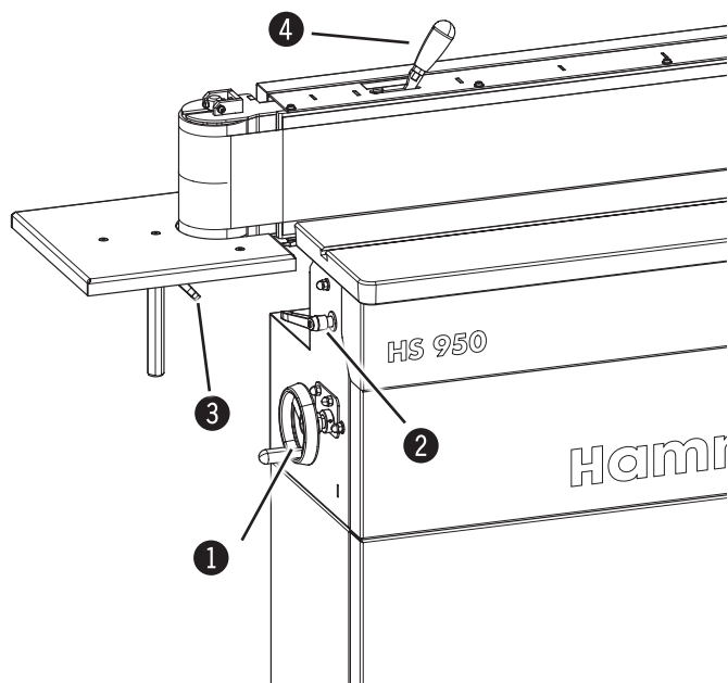
Fig. 5-5: Elementos de manejo e indicadores
