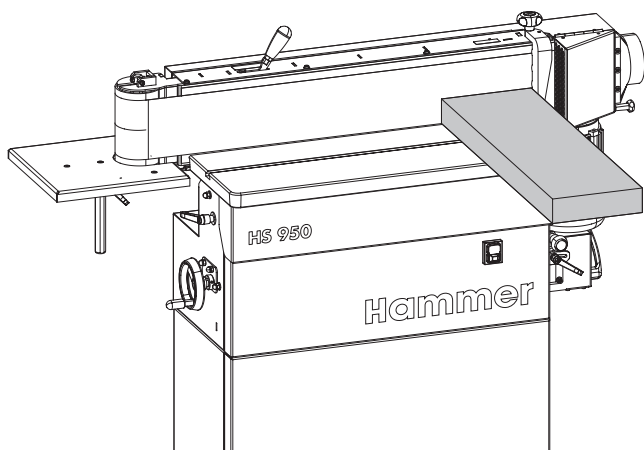
Fig. 9-4: El lijado en la parte delantera de la máquina
