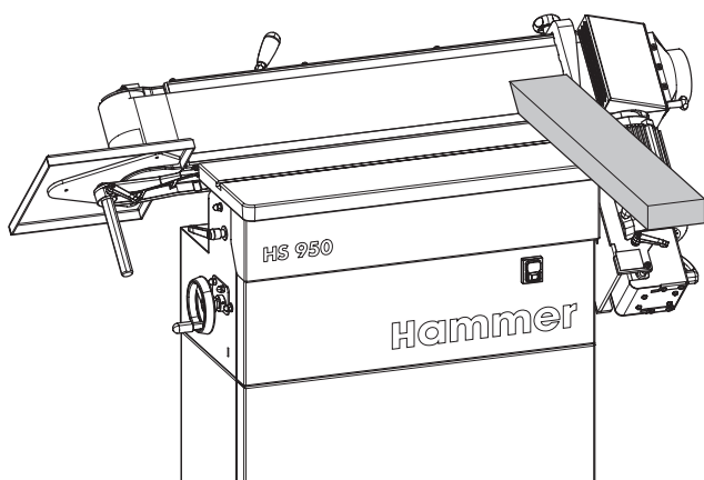
Fig. 9-5: El lijado con la unidad inclinada
