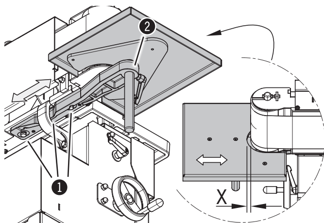
Fig. 7-11: Ajuste - Mesa de trabajo lateral
