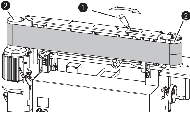
Fig. 8-1: Montaje banda de lijado
