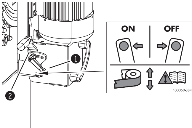
Fig. 8-5: Activar/desactivar la oscilación de la banda de lijado.
