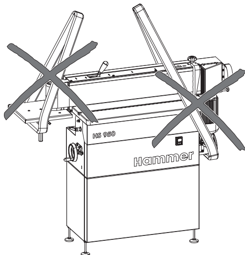
Fig. 6-2: Transporte con grúa
