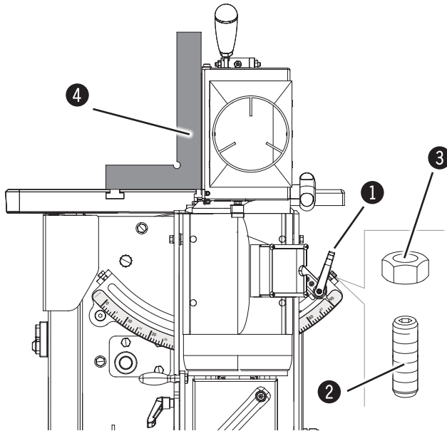
Fig. 11-2: Ajuste del ángulo - 90°
