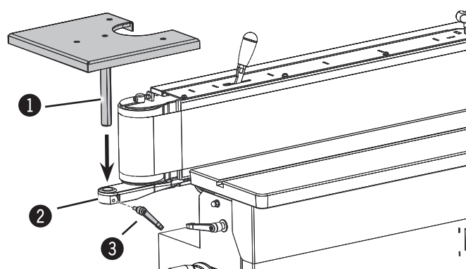
Fig. 7-10: Montaje - Tope de pieza
