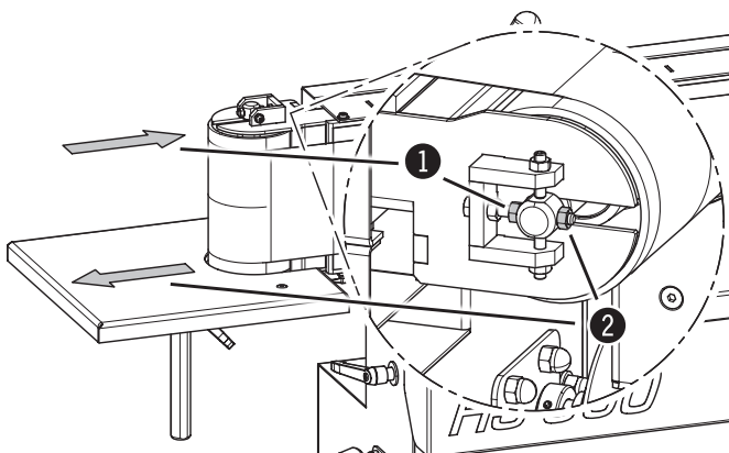
Fig. 8-2: Ajuste del recorrido de la banda
