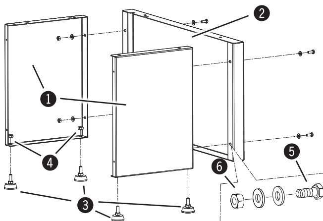
Fig. 7-4: Montar el armazón de la máquina
