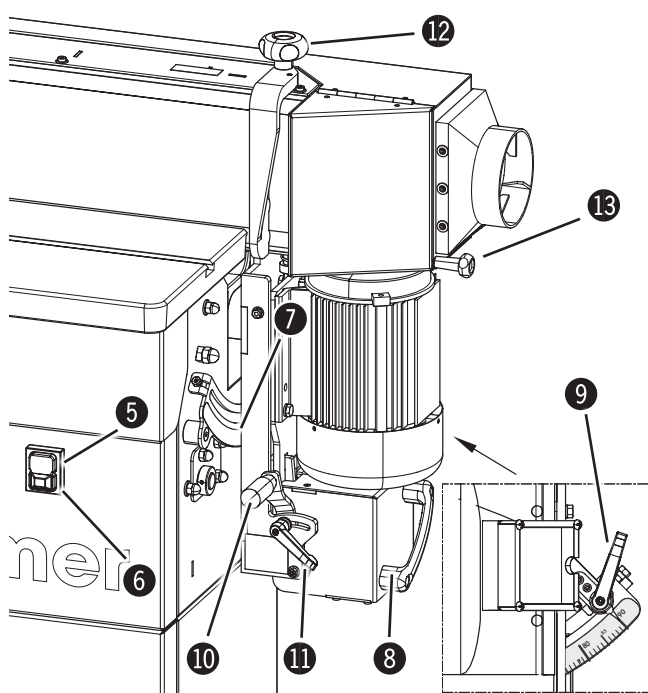
Fig. 5-6: Elementos de manejo e indicadores
