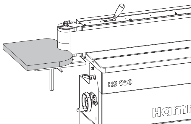
Fig. 9-8: Lijado en el rodillo
