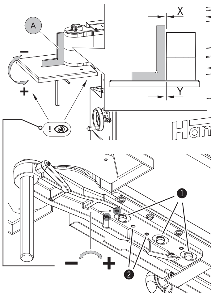
Ábra. 7-12: Beállítás - Szög A
