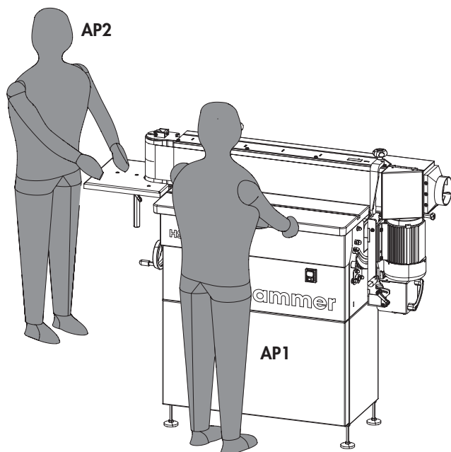
Ábra 9-3: Munkahely/munkapozíció
