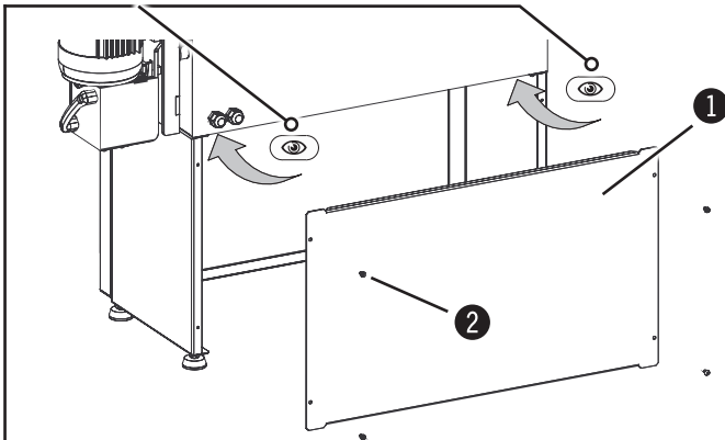
Ábra 10-1: Előkészület - Kenje meg a magasságbeállítót
