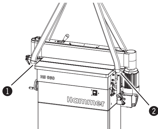
Ábra. 6-3: Szállítás daruval
