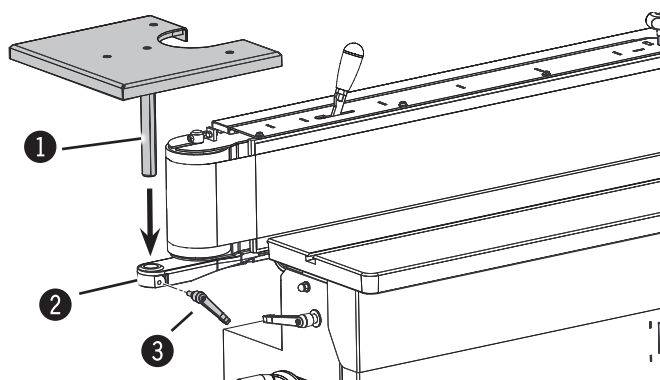
Ábra. 7-10: Szerelés - Munkadarab
