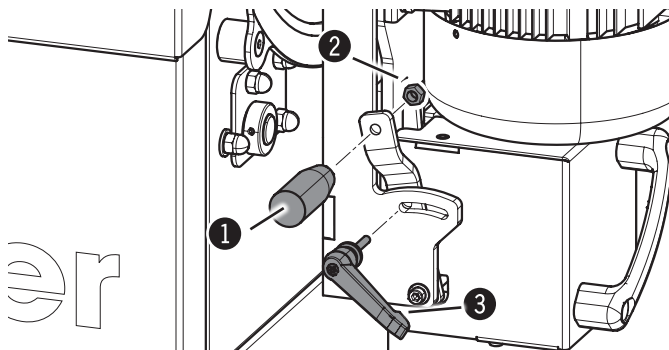
Ábra. 7-7: Szerelés - szabályozókar
