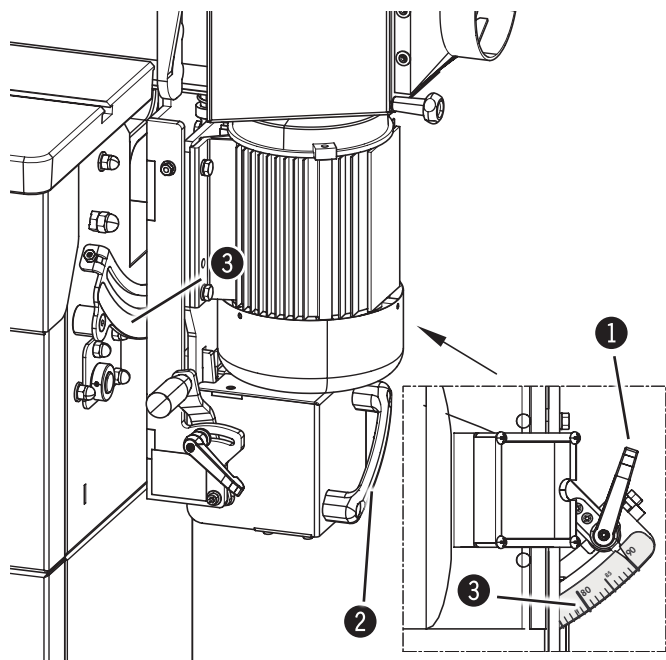
Ábra 8-4: A csiszolóegység szögbeállítása
