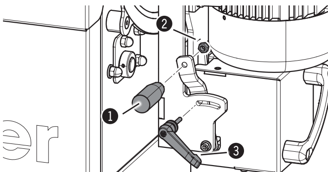
Abb. 7-7: Montage - Justiergriff
