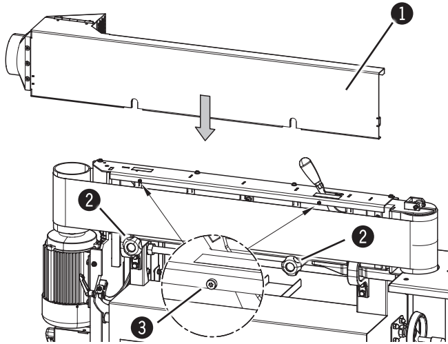
Abb. 7-8: Montage - Hintere Abdeckung Schleifband
