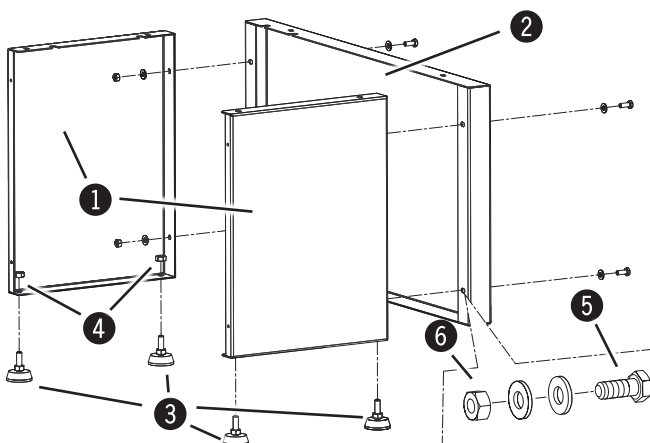
Abb. 7-4: Maschinengestell montieren
