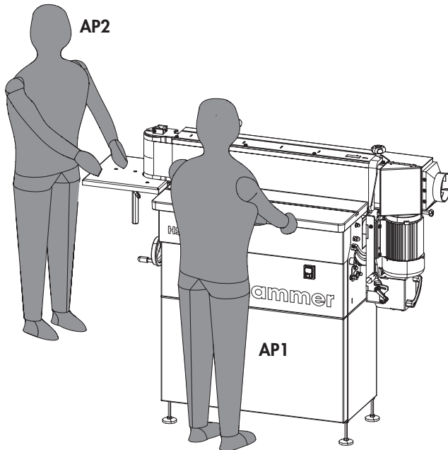
Abb. 9-3: Arbeitsplatz/Arbeitsposition
