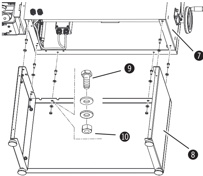
Abb. 7-5: Maschinengestell montieren
