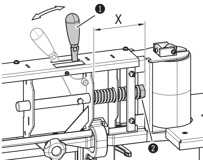
Abb. 11-1: Federspannung einstellen
